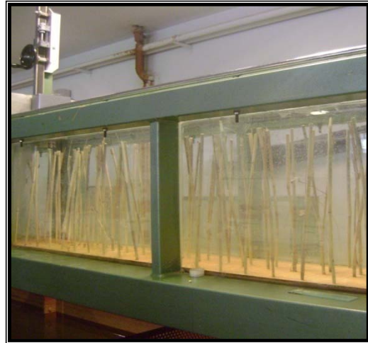
Fig.5. Roseau coupés et rangés à l'intérieur du canal
