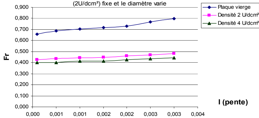
Fig. 16 Variation de nombre Fr en fonction la pente dans le cas où le diamètre (10mm) fixe et la densité varie
