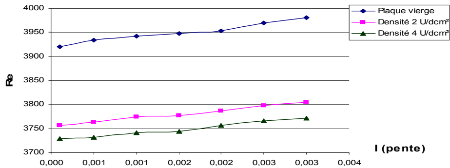
Fig. 14 Variation de nombre Re en fonction la pente dans le cas où le diamètre (7mm) fixe et la densité varie
