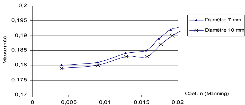
Fig. 8 Effet du diamètre de la tige du roseau sur la vitesse d'écoulement.(2 U/dcm 2 )
