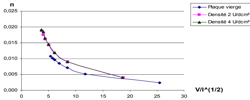
Fig. 10 Variation de coef. de rugosité n en fonction du terme V/I^{1/2} dans le cas où le diamètre fixe (7mm) et la densité variee
