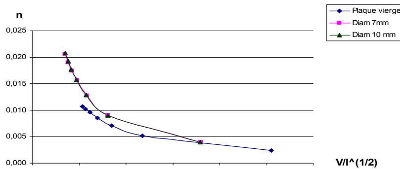
Fig. 13 Variation de coef. de rugosité n en fonction du terme V/I^{1/2} dans le cas où la densité fixe (4U/dcm²) et le diamètre varie
