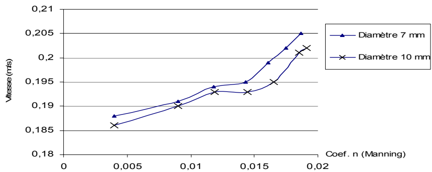
Fig. 8 Effet du diamètre de la tige du roseau sur la vitesse d'écoulement.(2 U/dcm 2 )
