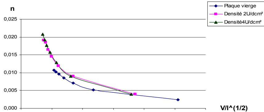
Fig. 12 Variation de coef. de rugosité n en fonction du terme V/I^{1/2} dans le cas où le diamètre fixe (10mm) et la densité variee
