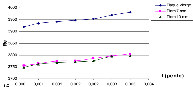
Fig. 15 Variation de nombre Re en fonction la pente dans le cas où la densité (2U/dcm²) fixe et le diamètre varie
