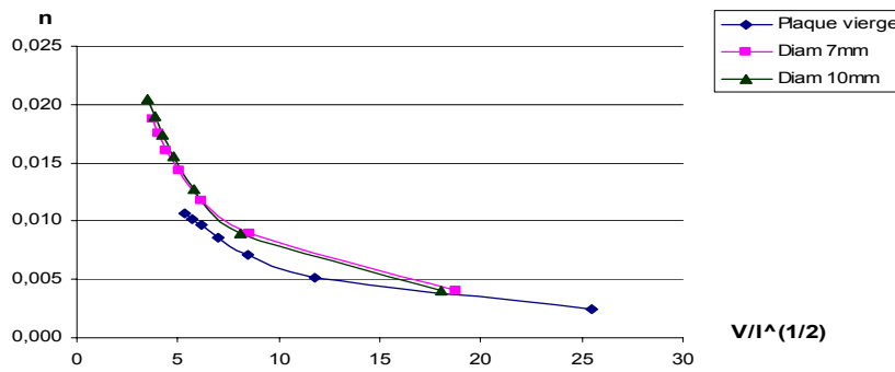
Fig. 11 Variation de coef. de rugosité n en fonction du terme V/I^{1/2} dans le cas où la densité fixe (2U/dcm²) et le diamètre varie
