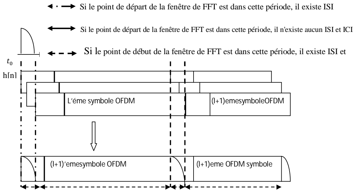
Figure II.8: Effet IES / ICI selon le point de départ de la fenêtre FFT.
