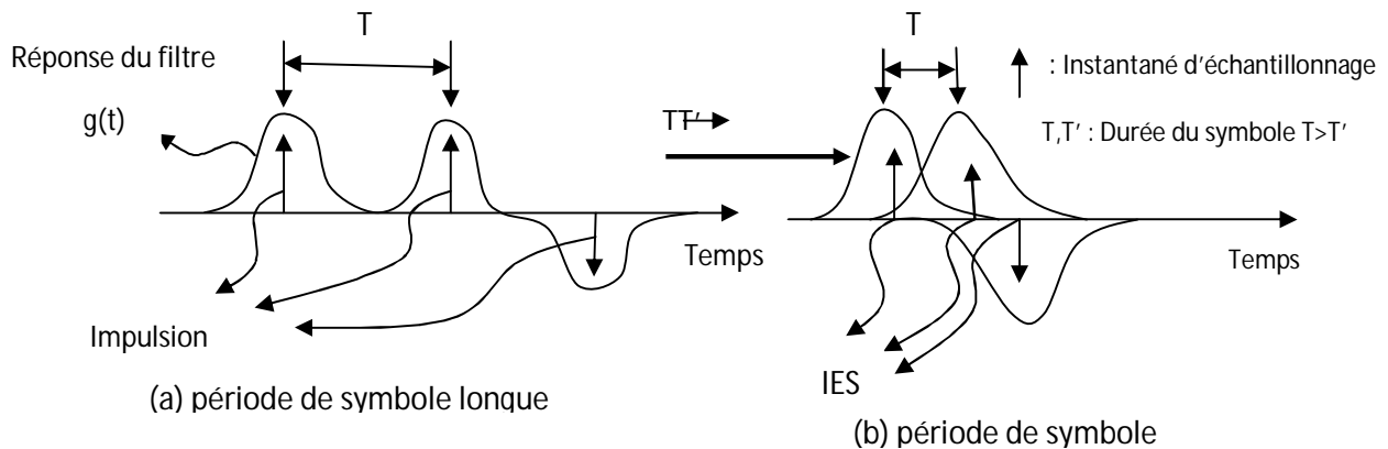
Figure II.2 : Interférence entre symbole (IES) et période de symbole.
