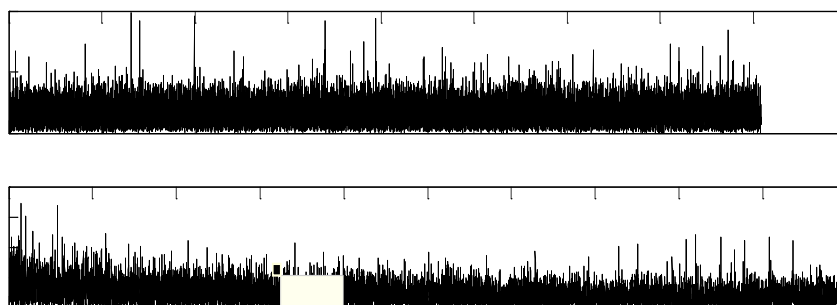
Fig. 3 Partie réelle de l'enveloppe complexe et son spectre d'enveloppe
