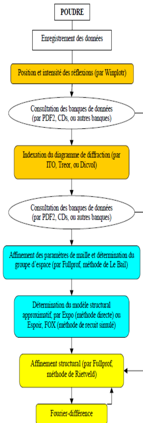
Figure 1a : Algorithme de la résolution structurale ab initio pour une poudre
