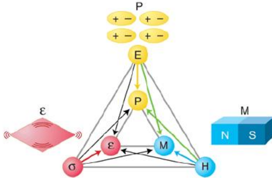
Fig.II.1: Relations de couplages dans les multiferroïques.
