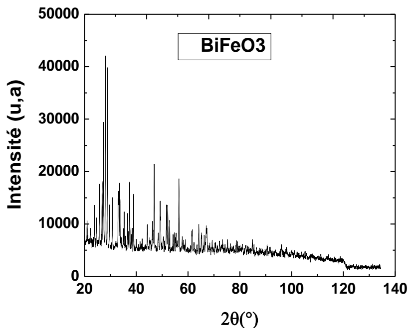
Fig.III.3 : Diagramme de diffraction X de \text{BiFeO}_3
