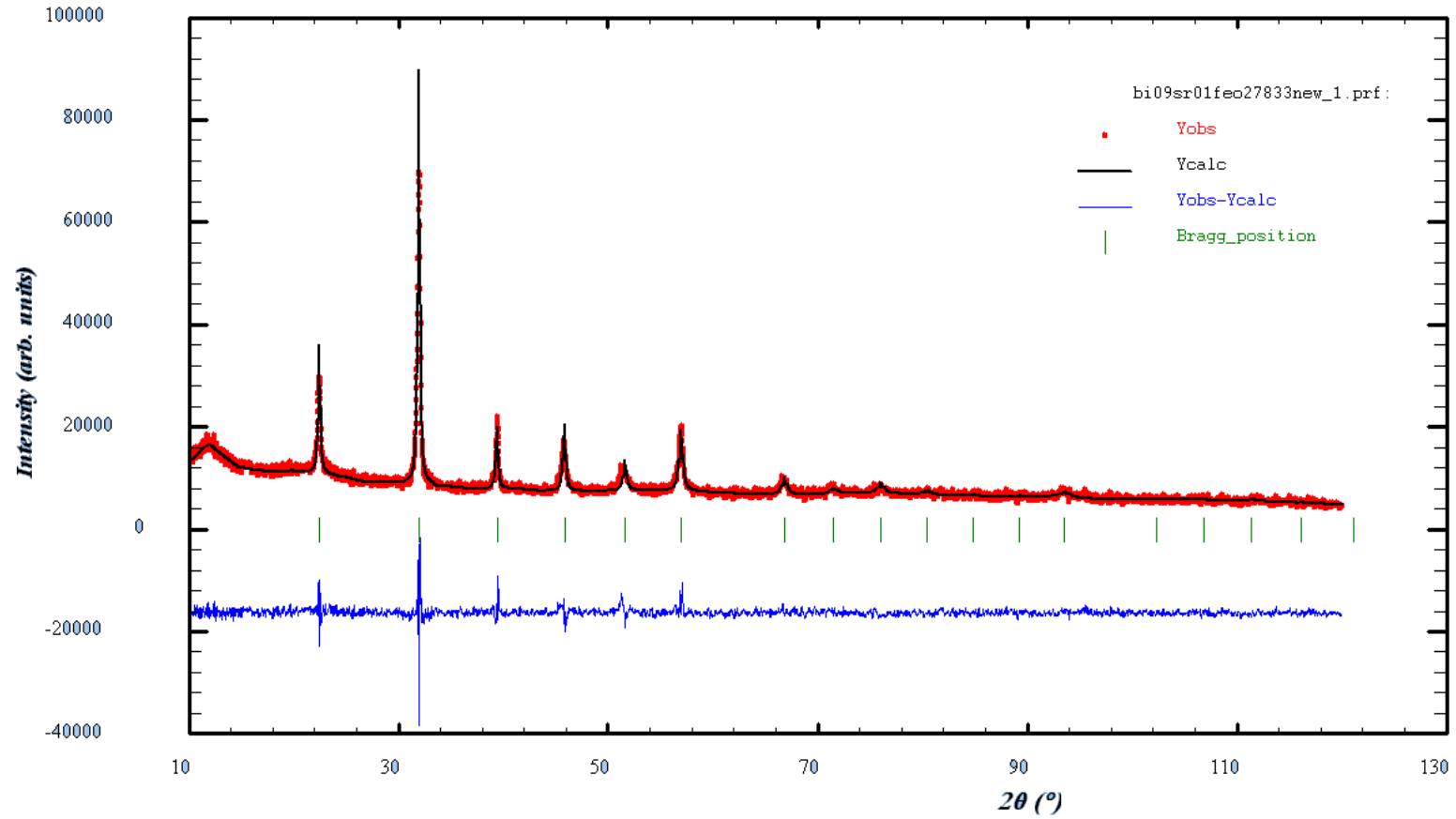
Fig. III.7 : Résultats d'affinement du Bi 0.9 Sr 0.1 FeO 3 par la méthode de Rietveld
