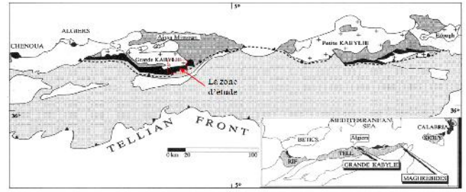
Fig.2. Schéma structural simplifié de la zone centrale de la chaîne des Maghrébides illustrant la position de la dorsale calcaire (en noir) [8]
