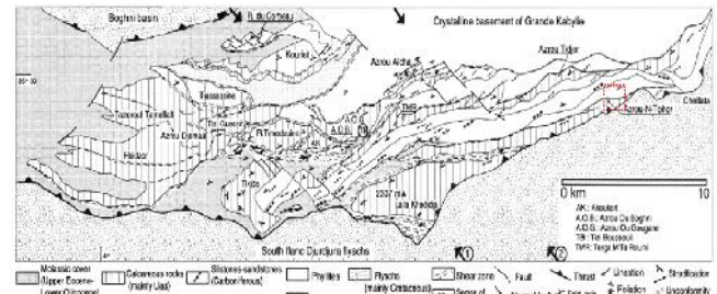
Fig. 3. Schéma structural de la dorsale calcaire du Djurdjura (Grande Kabylie, Algérie) ([4], [2], [9]).
