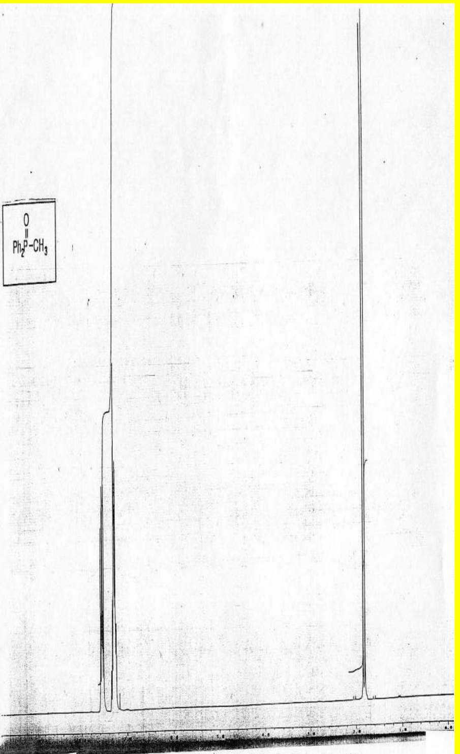
Figure (6) Spectre RMN 1 H de l'oxyde de méthyl diphenyl phosphine
