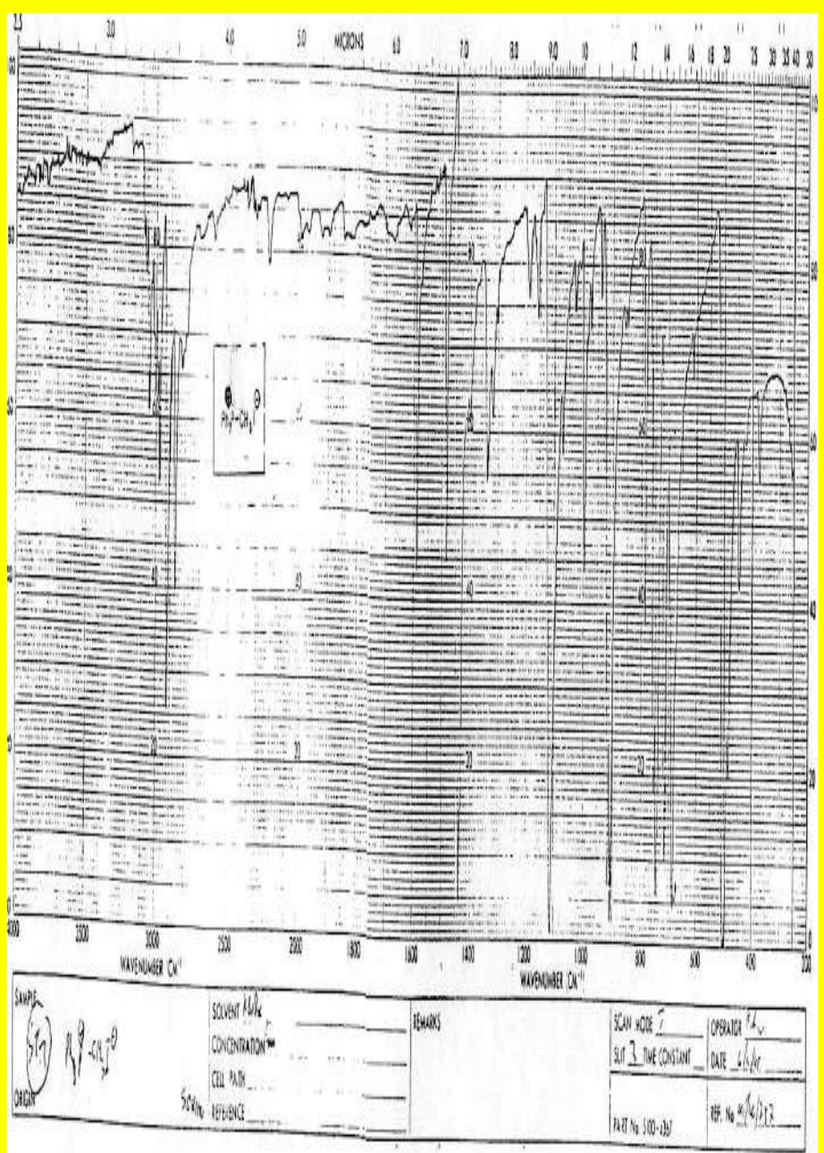
Figure (1) Spectre I.R. de l'iodure de méthyl diphenyl phosphonium
