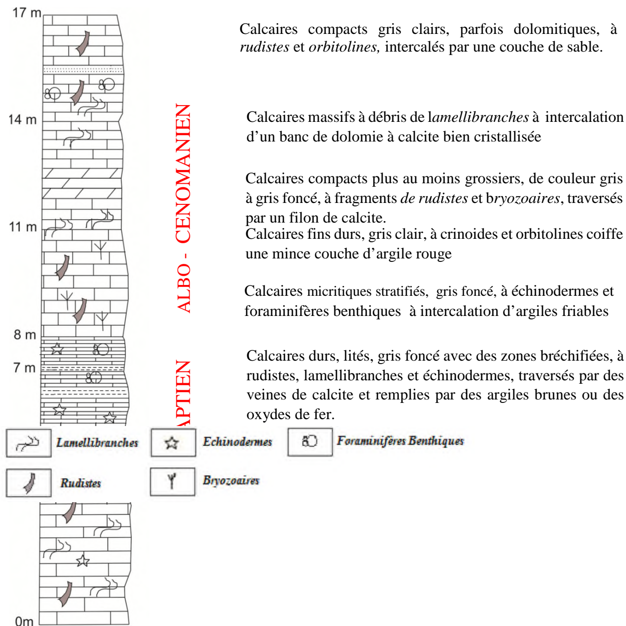
Fig. 2. Coupe lithologique des formations carbonatées de la zone de la Mine.
