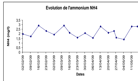
Fig.10. Evolution de la NH 4 à la sortie
