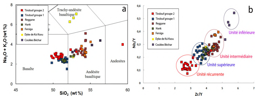
Figure 3. a) Diagramme silice-alcalins (TAS) des dolérites du Sud-Ouest algérien. Les analyses ont été recalculées en base anhydre et normalisées à 100 %. b) Variation des rapports Nb/Y et Zr/Y des dolérites du Sud-Ouest algérien.
