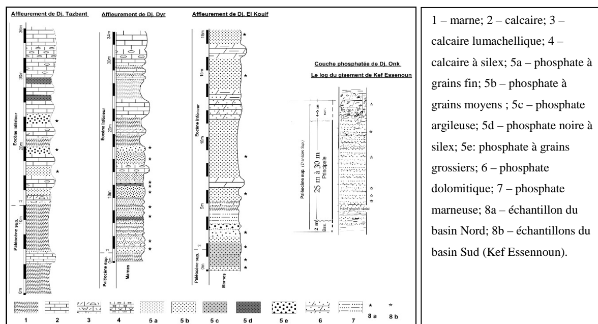
Fig. 2. Logs lithologiques échantillonnés pour la présente étude.
