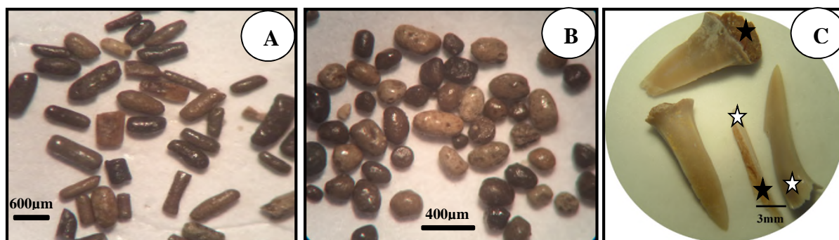
Fig. 3 : Particules phosphatées séparées. A) Coprolithes ; B) Pellets ; C) Dents de poissons : Dentine (partie interne: étoiles remplies), Email (partie externe : étoiles vides).
