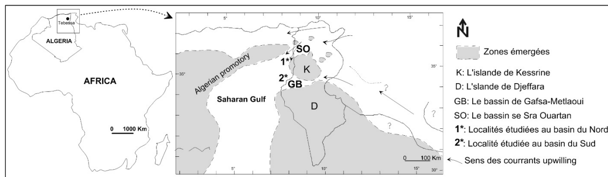
Fig. 1 : Localisation des bassins phosphatés et paléogéographie durant le Paléocène- Eocène Inférieur [6-8 ; 24 ; 26-27].
