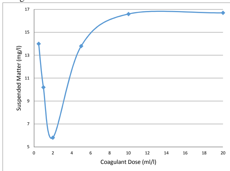
Figure 2 : Effet de la dose de cactus sur la matière en suspension
