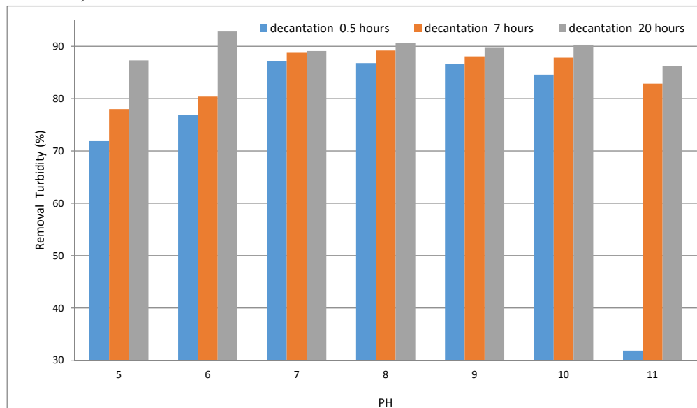
Figure 3: Effet du temps de décantation sur la réduction de la turbidité
