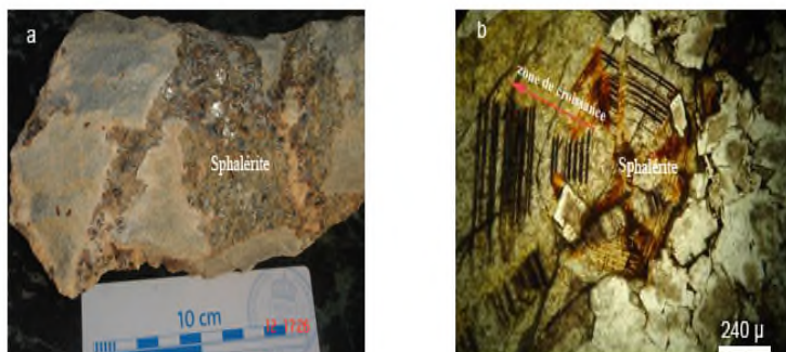
Aspect macroscopique (a) et microscopique (b) de la sphalérite
