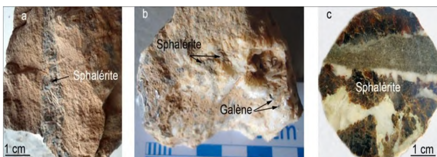
Exemple de quelques textures de minerais du gisement de Merouana
