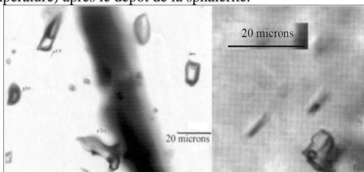
Inclusions fluides aqueuses biphasées dans la sphalérite de Mérouana
