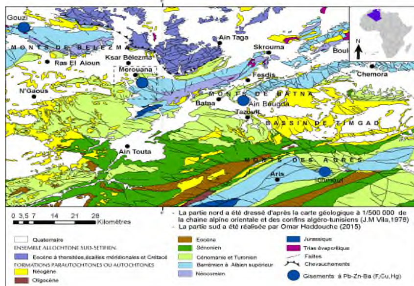
Carte géologique de Merouana et des régions voisines
