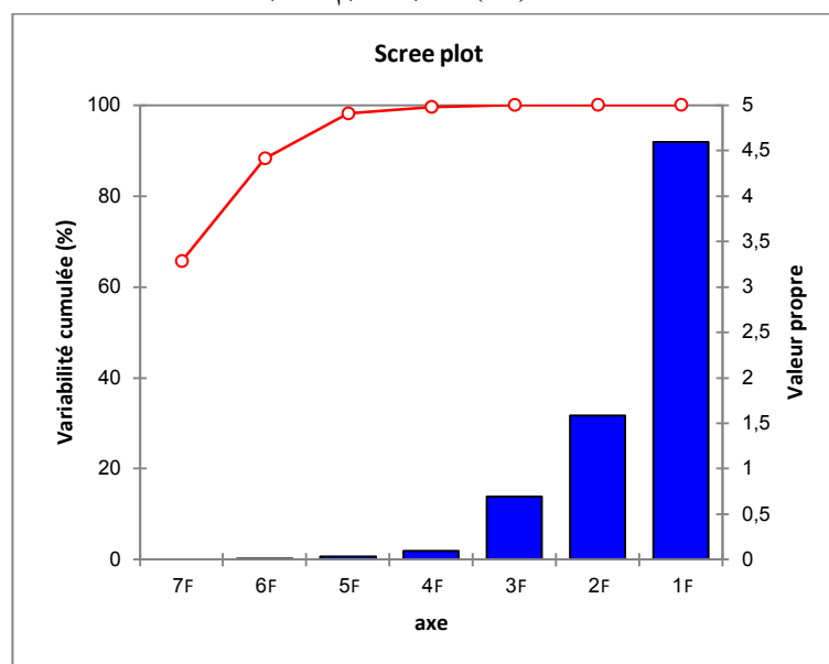
الشكل (02): تمثيل القيم الذاتية
