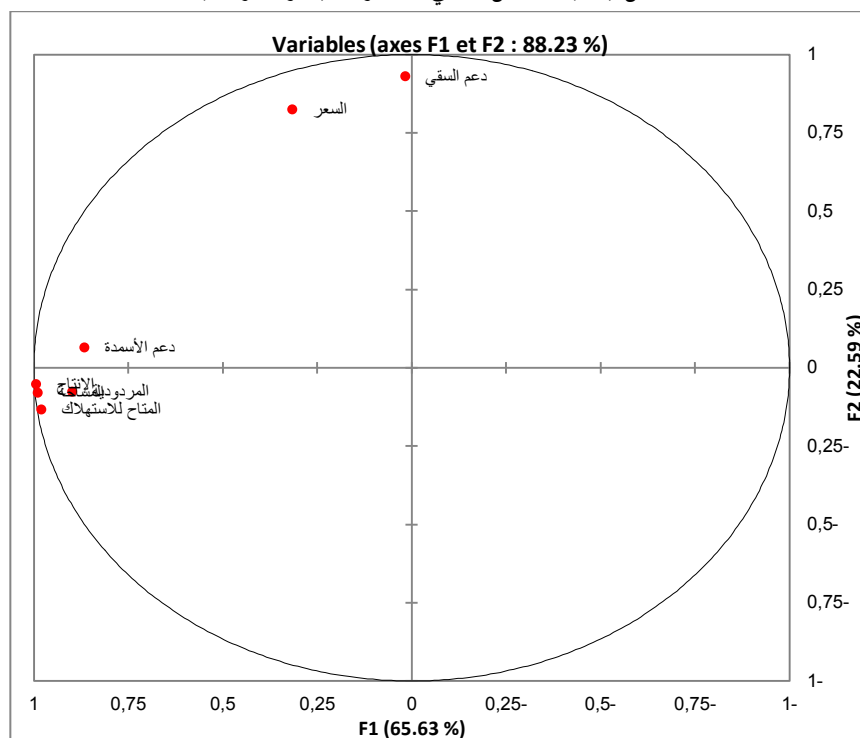
الشكل (03): التمثيل البياني للمتغيرات (دائرة الارتباط)
