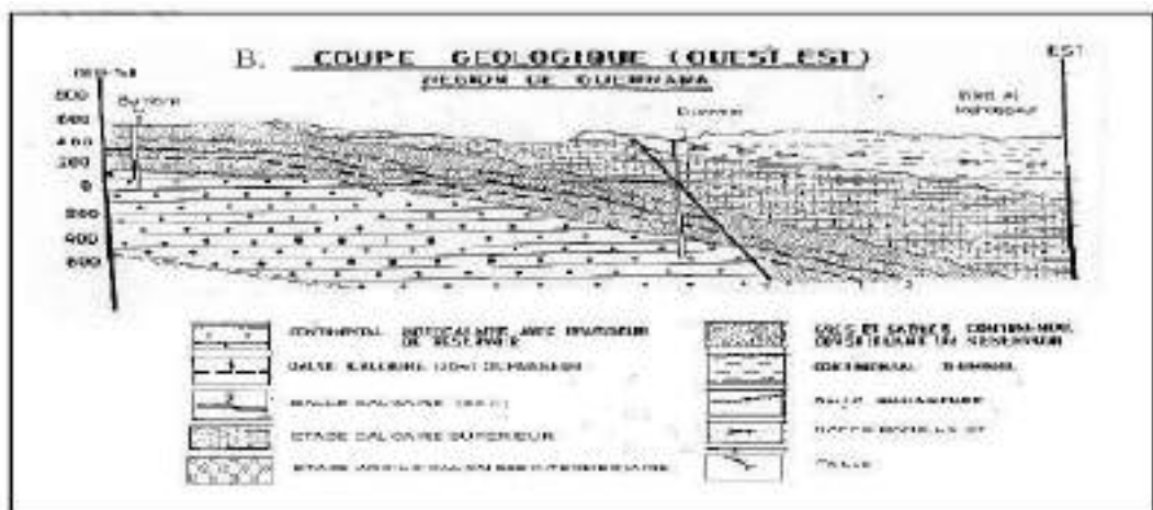
Figure 06: Coupe géologique de Guerrara (S.C.G, 1952, HADJ SAID.S et al, 2008)
