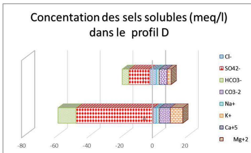
Figure 24 : Profil ionique du profil D
