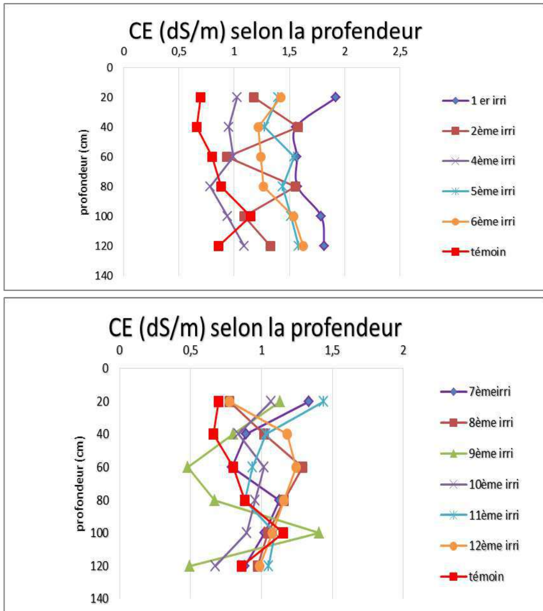
Figure 27 : Evolution de la CE moyenne (dS/m) en fonction de la profondeur des profils (Site A) (Annexe 9)
