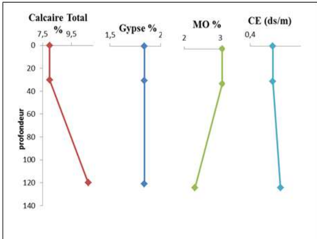
Figure 17. Profils calcaires, matière organique, gypse et de CE du profil B
