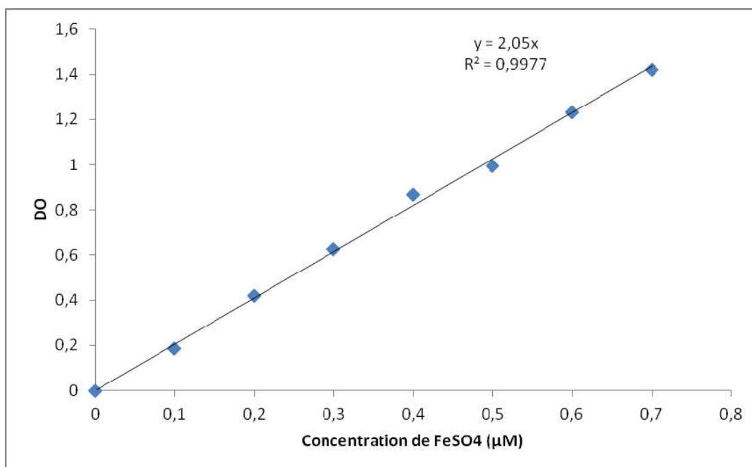
Annexe 8 : Courbe d'étalonnage de \text{FeSO}_4 pour le test FRAP.
