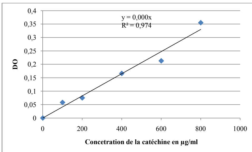
Annexe 4 : Courbe d'étalonnage de la catéchine.
