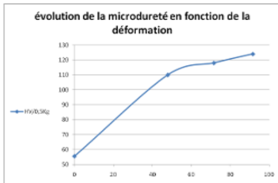
Figure 2 : Evolution de la valeur moyenne de la microdureté en fonction du taux de r duction.
