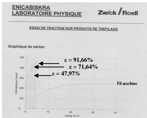
Figure 3. Graphique de la s rie des essais de traction apr s avant recuit.
