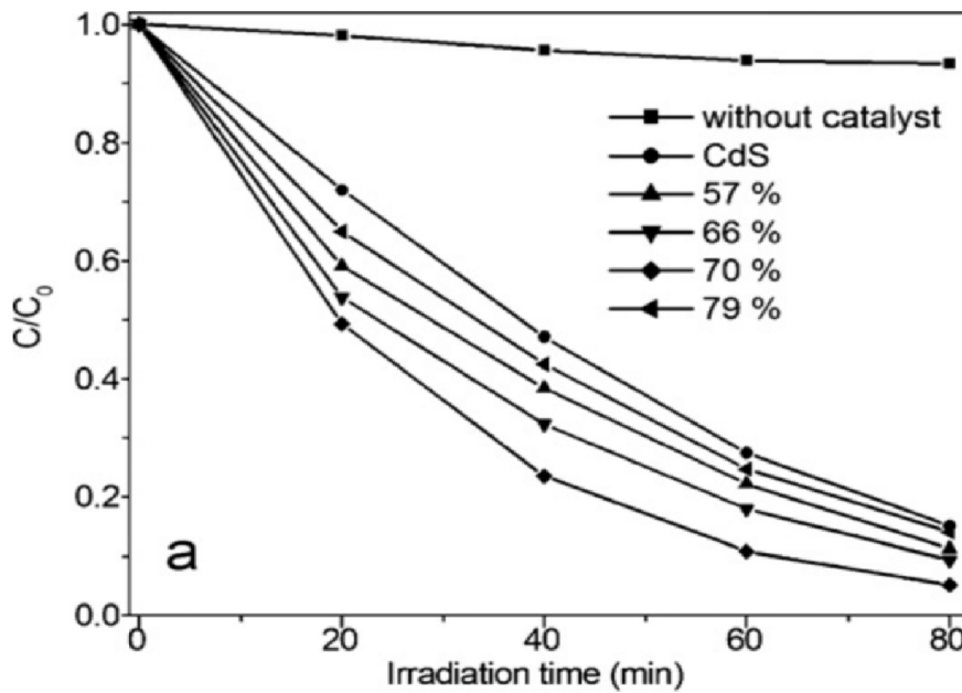
الشكل (6-III): التفكك الضوئي لـ Rh-B المحفز بواسطة CdS و CdS/GR باستعمال كميات مختلفة من CdS تحت اشعة الضوء المرئي .
