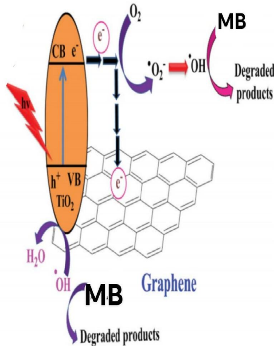
الشكل (4-III): آلية التحفيز الضوئي للمركب \text{TiO}_2/\text{GR} [8]
