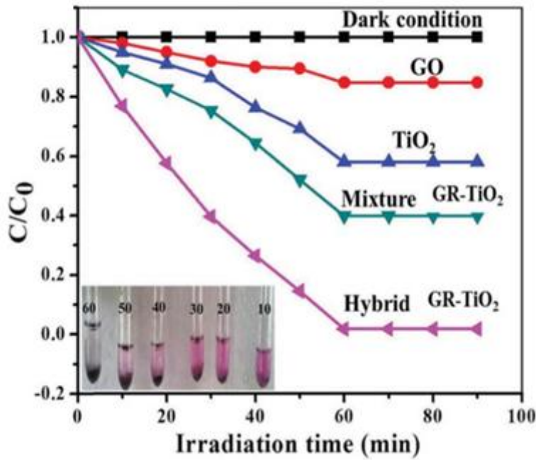
الشكل (2-III):دراسات المقارنة لتفكك Rh-B في محفزات مختلفة
