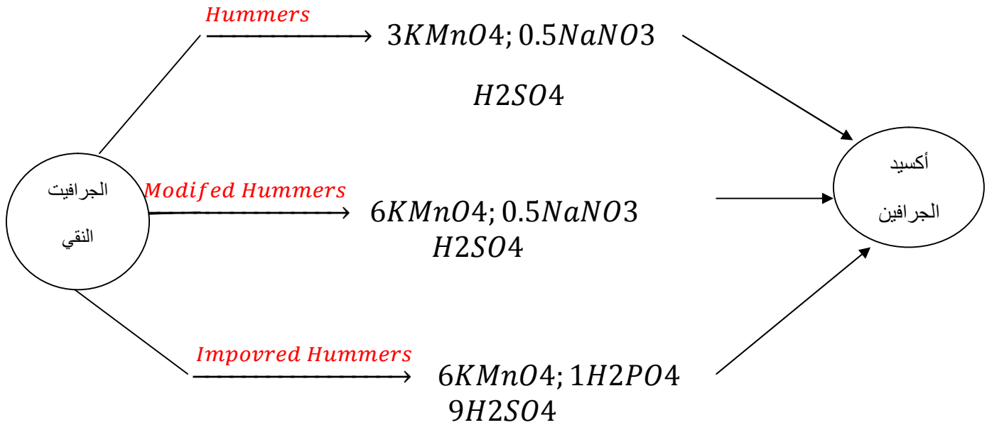
الشكل (II-9): بعض الطرق المستخدمة في اصطناع أكسيد الجرافين [1]
