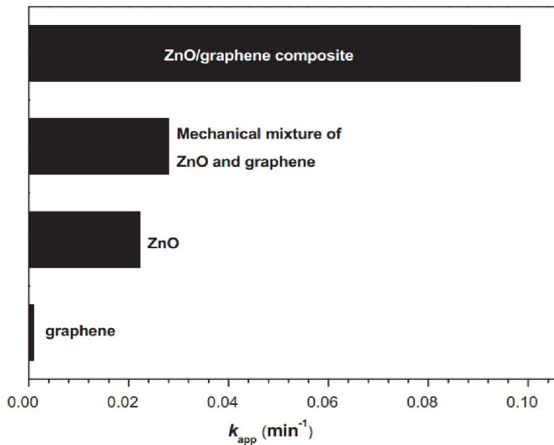
الشكل (5-III): ثابت معدل التفاعل لتفكك MB للمركبات ZnO النقي، خليط ZnO /GR، المركب المهجن ZnO /GR .
