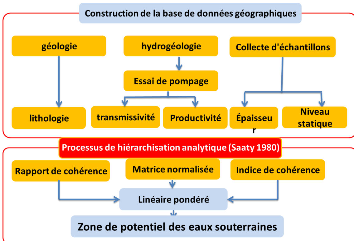
Figure 47: Organigramme illustrant les différentes étapes de l'étude
