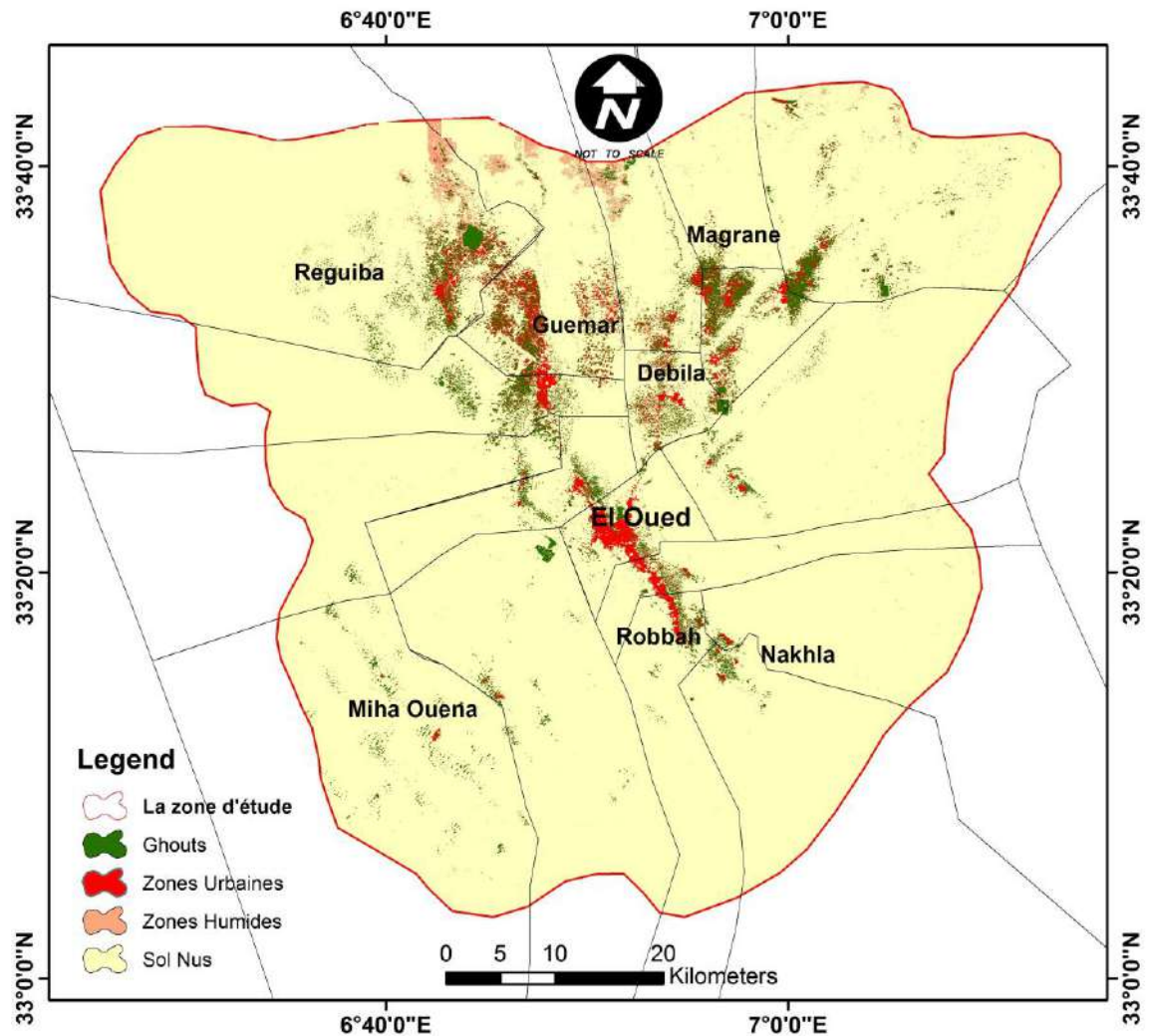
Figure 06: carte d'occupation du sol de la région d'étude (2000)
