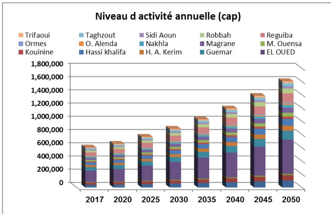
Figure 99. Evolution de la population dans la zone d'étude Scénario 1 : Scénario de référence (2018-2050)
