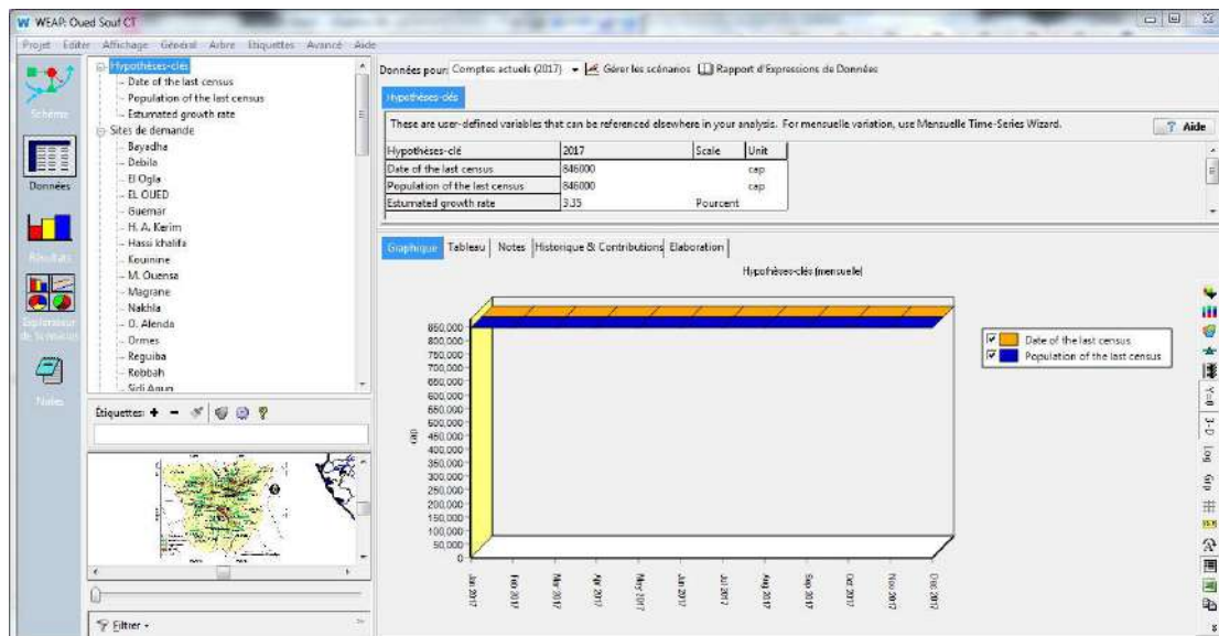
Figure 97. Fenêtre montrant les hypothèses clés et le compte courant.
