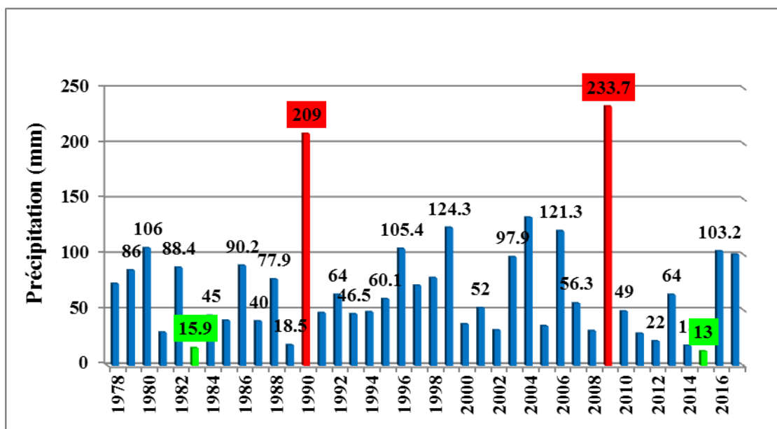
Figure 09: Histogramme des variations annuelles des précipitations.
