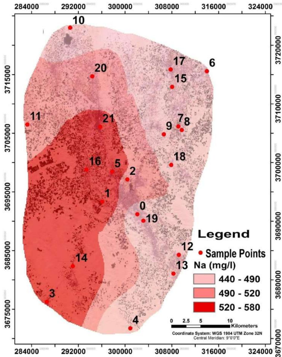
Figure 60: Carte de distribution spatiale de sodium
