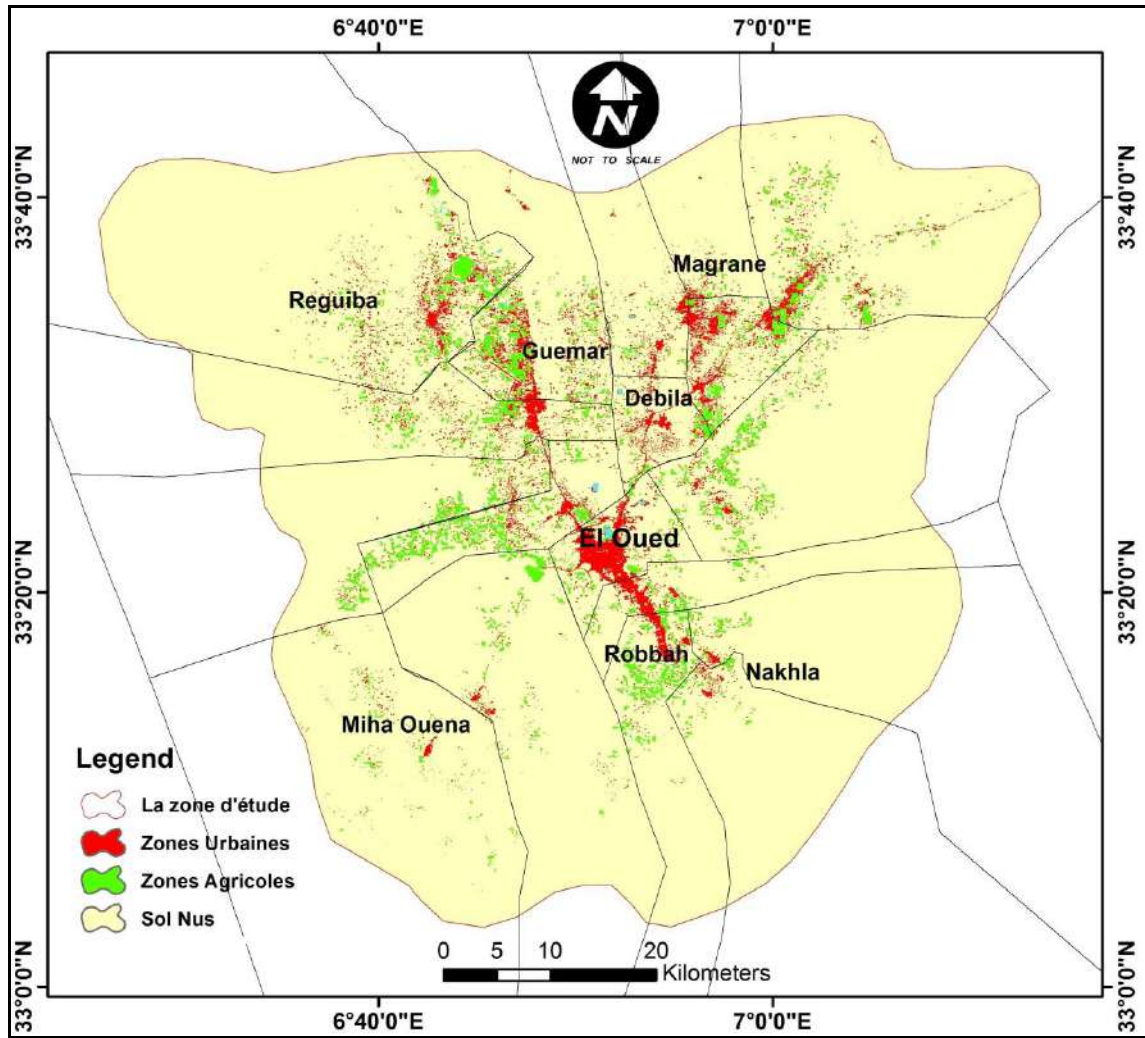
Figure 07: carte d'occupation de sol de la région d'étude (2010)
