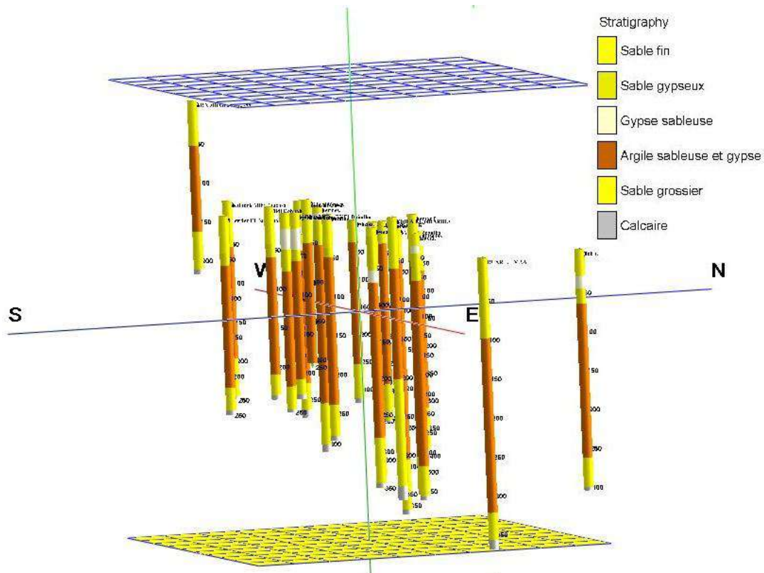
Figure 22: Localisation des 26 logs de forages sélectionnés. (Représentation de la stratigraphie en 3D)
