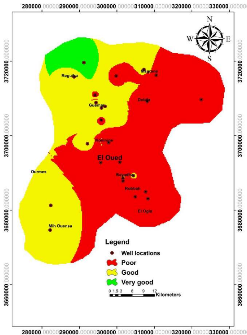
Figure 52: Zones potentielles d'eaux souterraines à Oued Souf
