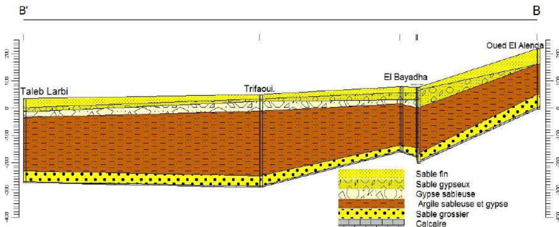
Figure 24: Coupes litho-stratigraphiques N°01
