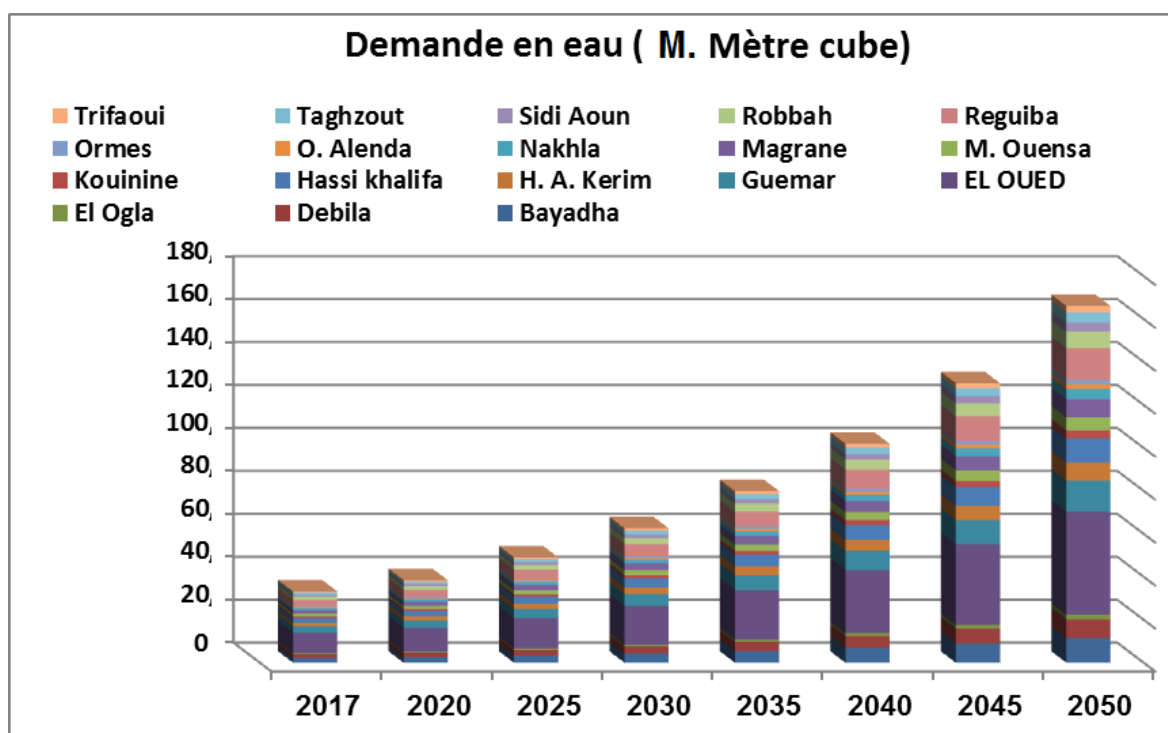
Figure 106. Evolution de la demande en eau - Scénario 2 : Fort accroissement de la populaion (2018-2050)-
