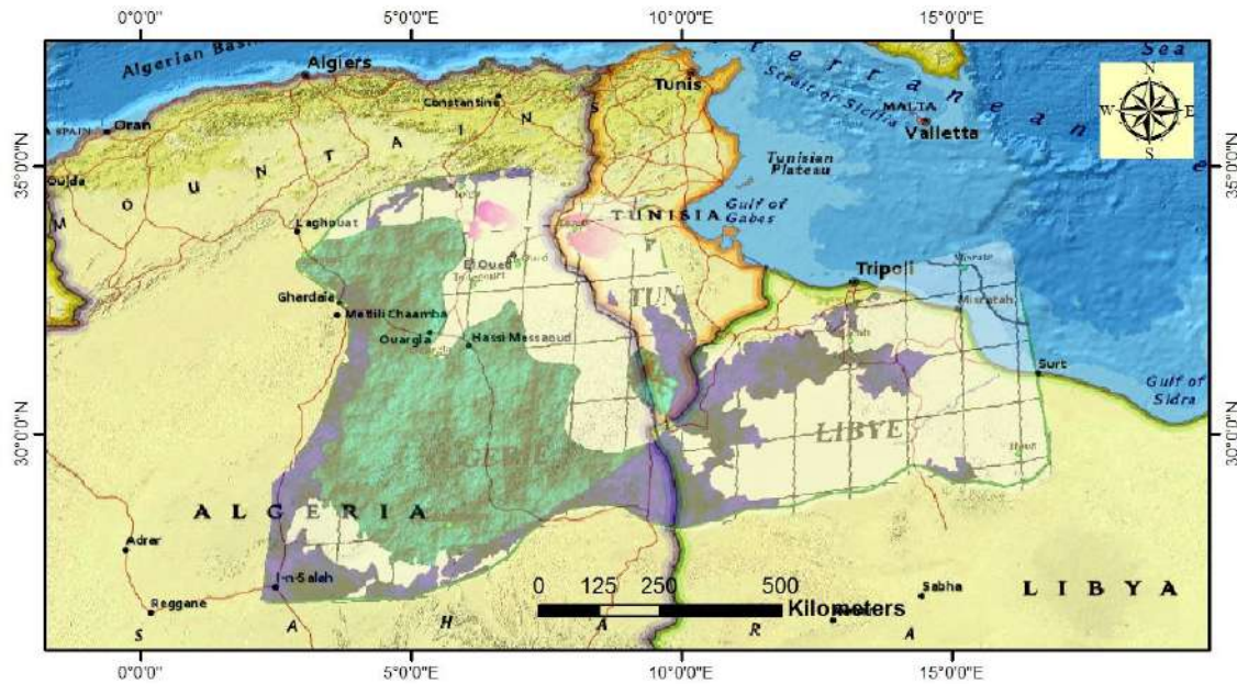
Figure 39: Les zones d'alimentation de CT (Baba SY, 2005). Modifier
