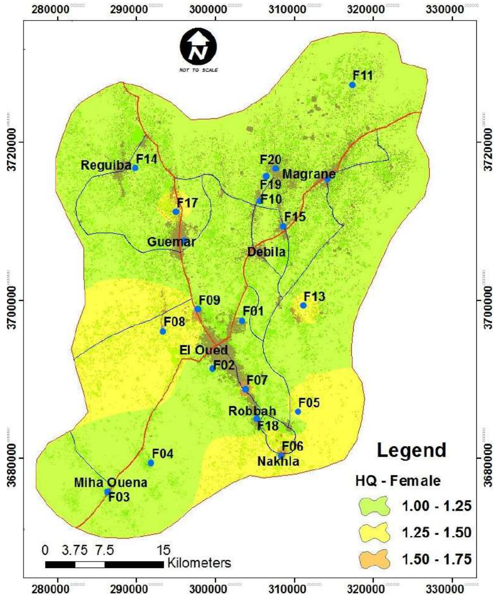
Figure 90: Distribution spatiale du risque pour la santé dû à la contamination par le fluorure dans les eaux souterraines (Femmes)
