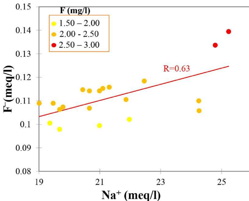
Figure 83: Relation entre F - et Na + .
