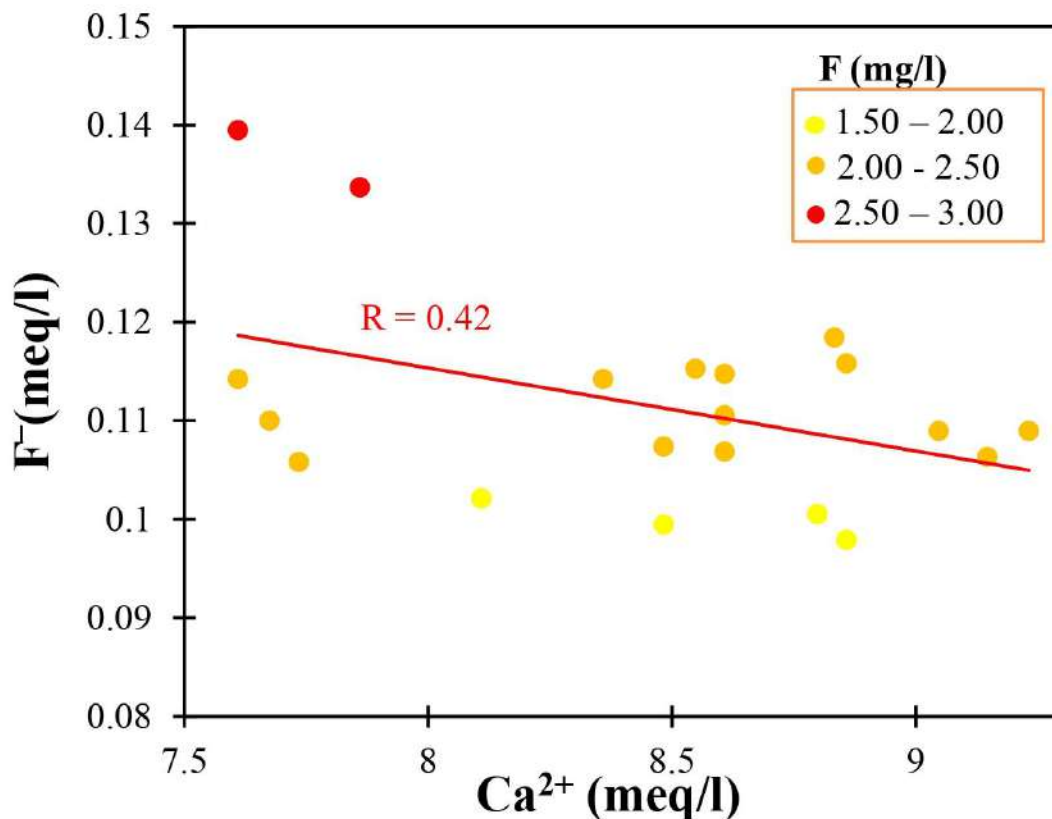
Figure 80: Relation entre F - et Ca 2+
