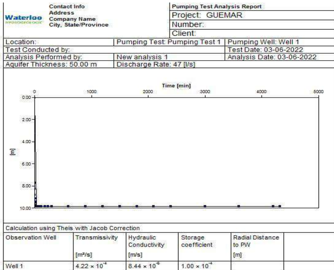
Figure 43: Essai de pompage longue durée à Guemar
