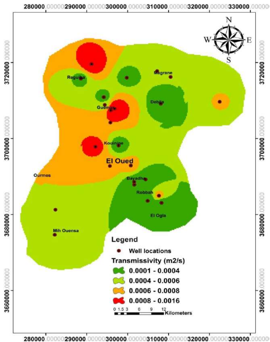
Figure 49: Distribution spatiale de la transmissivité de l'aquifère CT.
