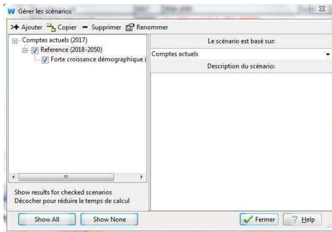
Figure 98. Création des scénarios.
