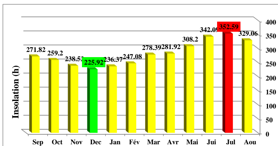
Figure 16 : Insolation de la région du Souf (1997-2009).
