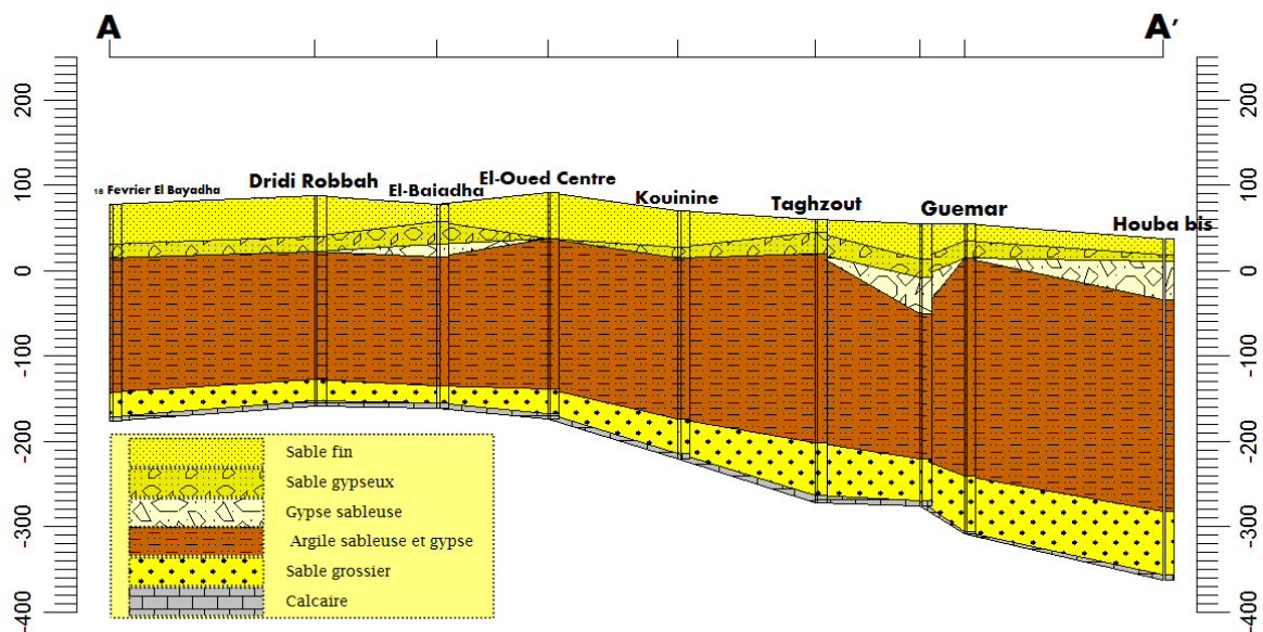
Figure 25: Coupes litho-stratigraphiques N°01
