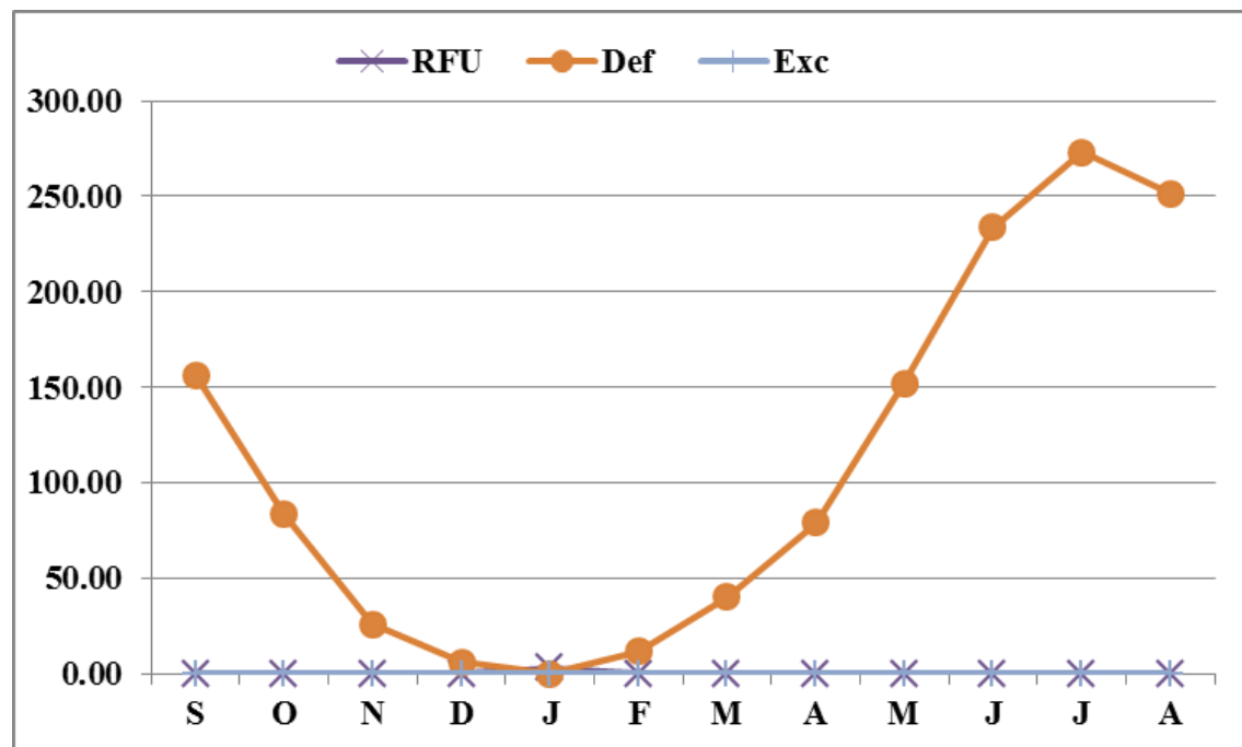
Figure 18: Etat de réserve facilement utilisable et le déficit agricole dans la région d'El-Oued.
