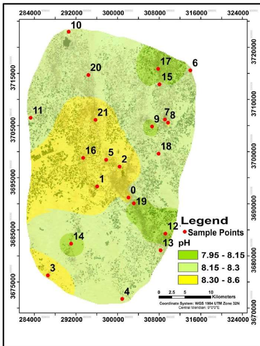
Figure 55: Carte de distribution spatiale de potentiel hydrogène
