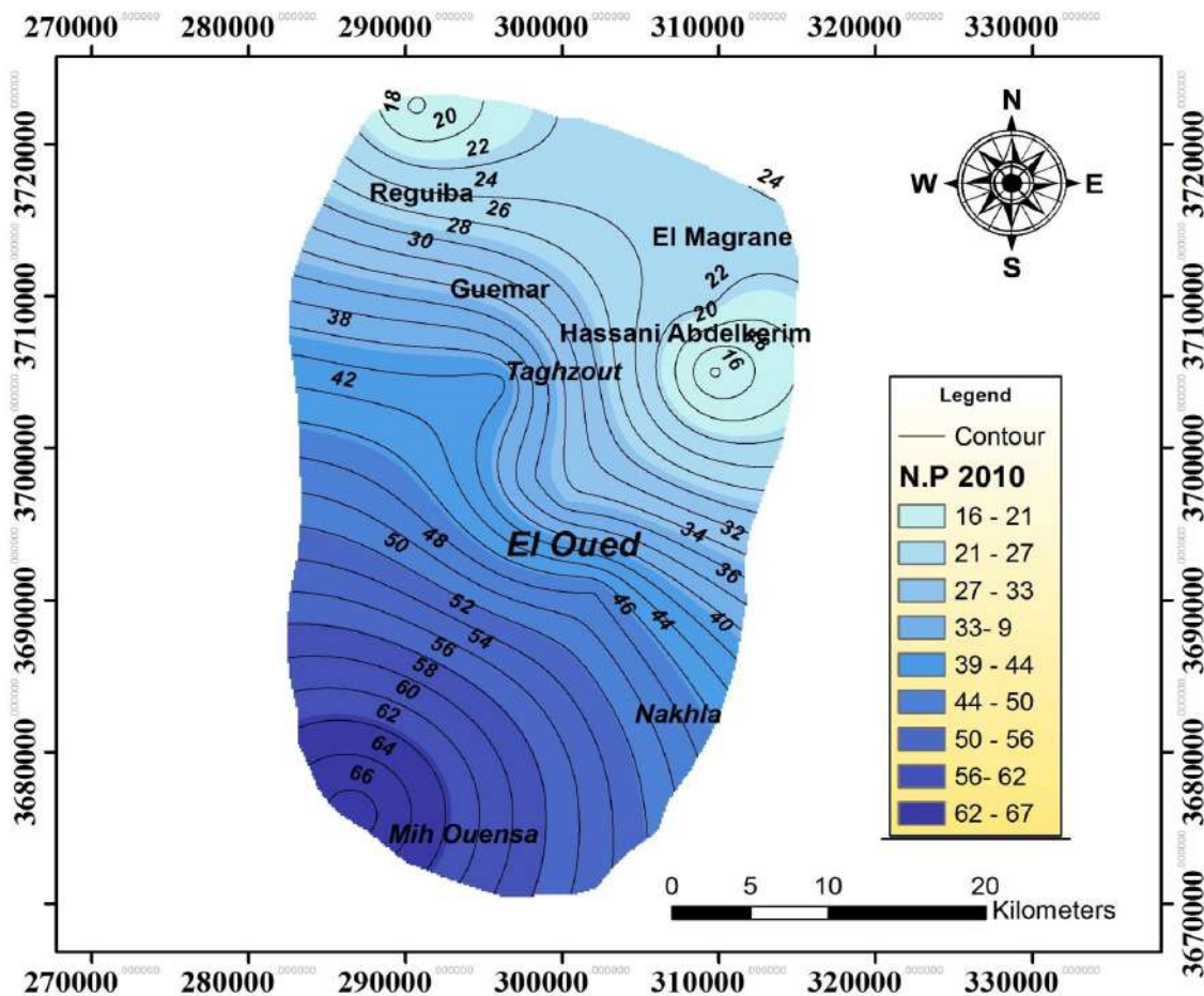
Figure 36: Carte du niveau piézométrique des eaux souterraines des aquifères du CT (mars 2010).
