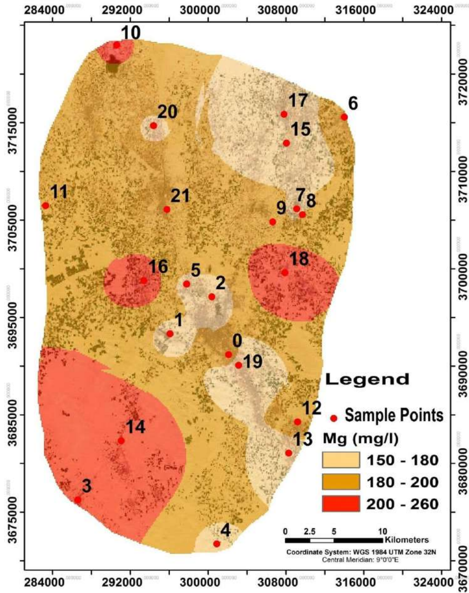
Figure 58: Carte de distribution spatiale du magnésium
