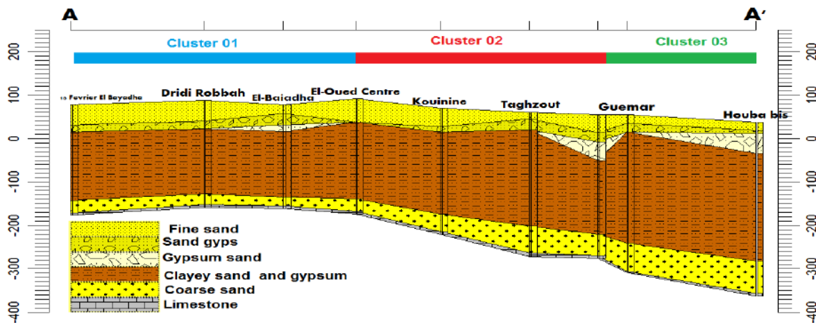
Figure 77: Distribution spatiale du CE pour les clusters d'eau souterraine.
