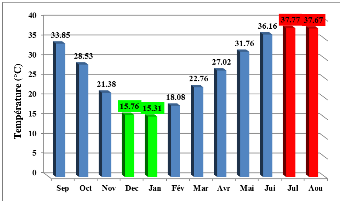
Figure 11: Histogramme des températures moyennes mensuelles (1978-2017).
