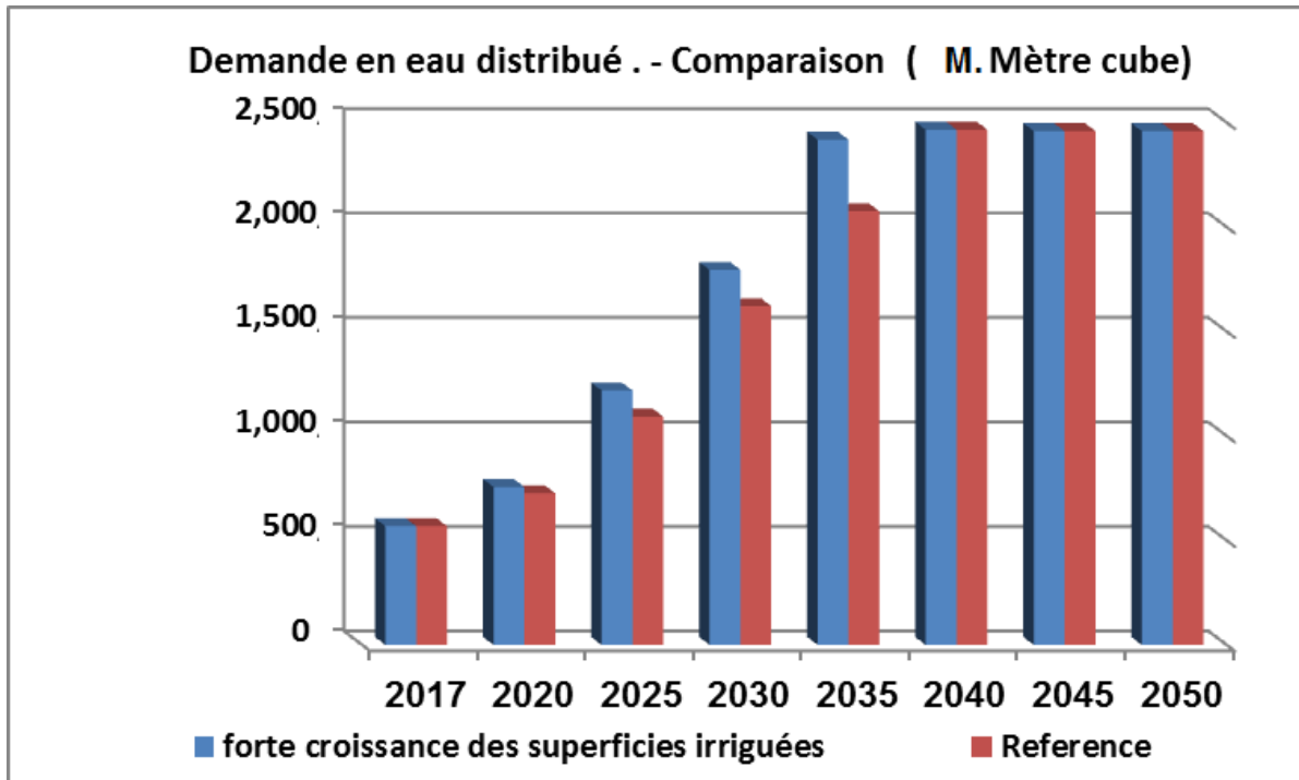
Figure 116. Evolution de l'eau distribué . - Comparaison avec le scénarios (2018-2050)-
