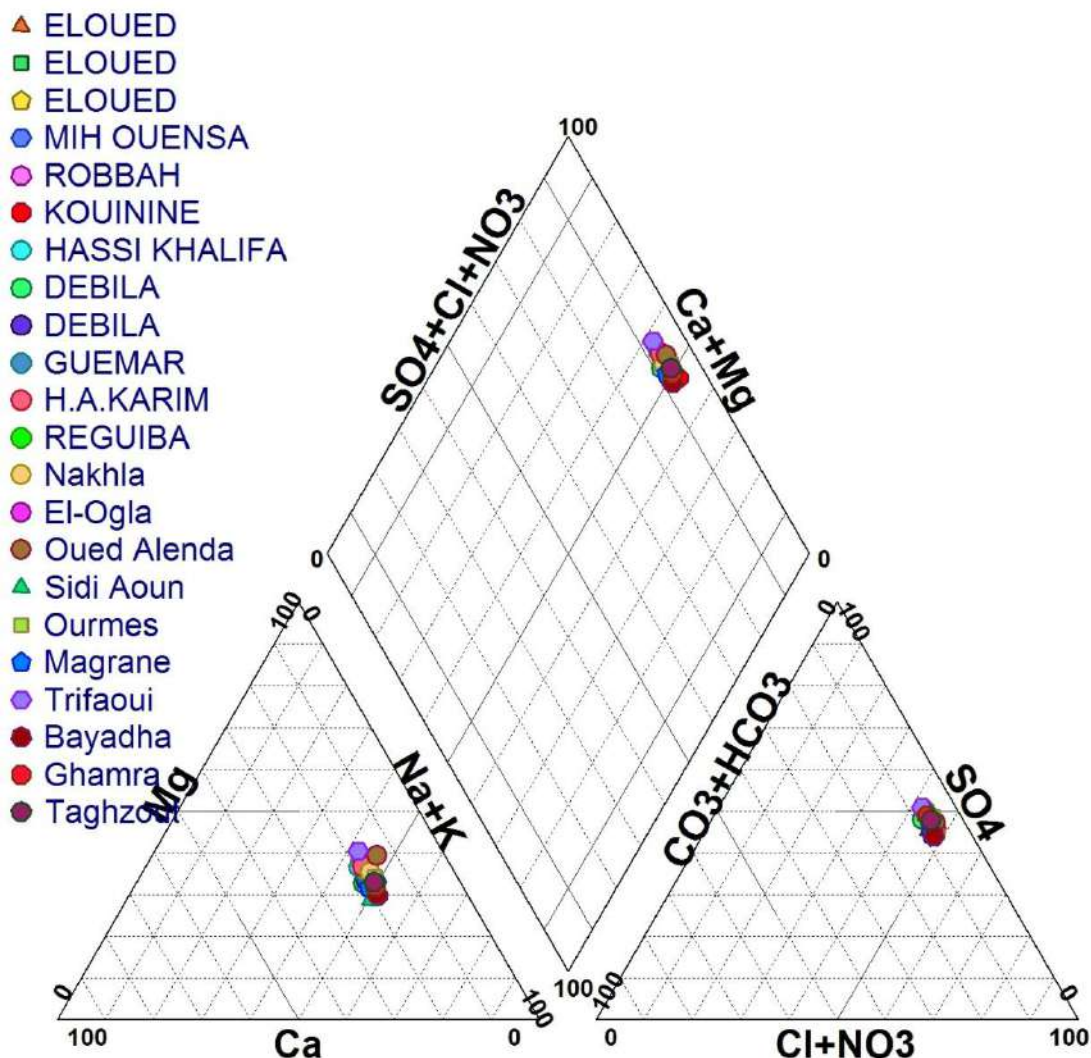
Figure 54 Faciès chimique des eaux souterraines
