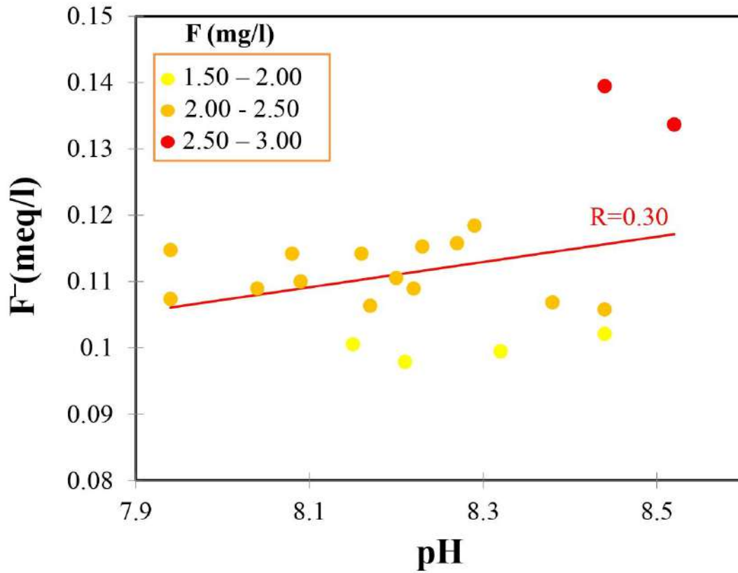
Figure 81: Relation entre F - et le pH
