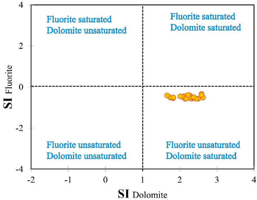
Figure 87: Diagrammes de fluorite (SI)vs dolomite (SI)
