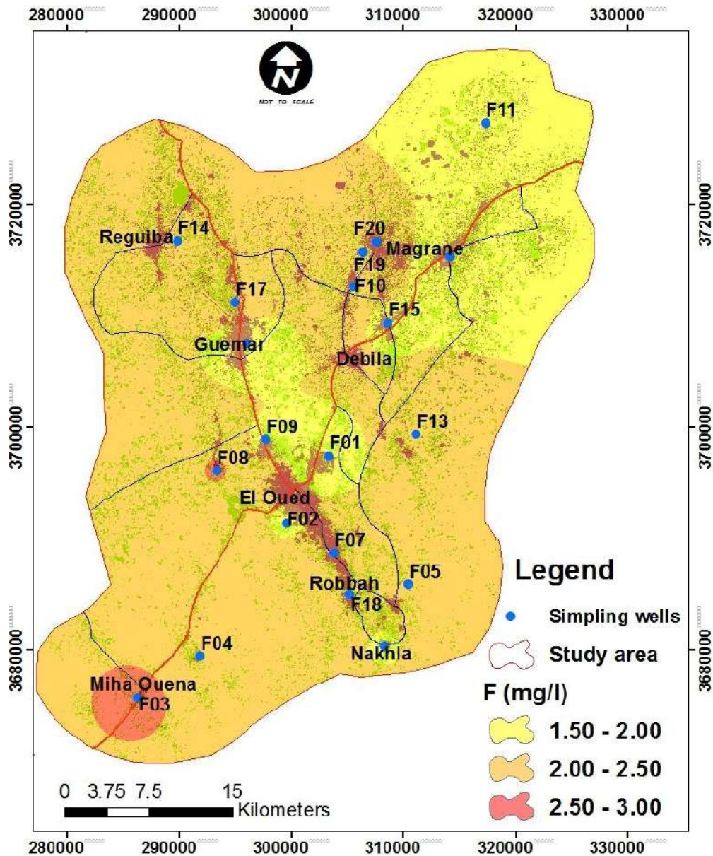
Figure 79 Distribution spatiale du fluorure dans les eaux souterraines
