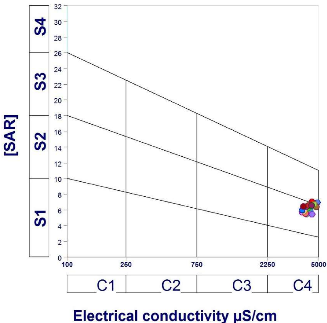
Figure 67: Représentation graphique de la classification de l'eau pour usage d'irrigation, diagramme USSS).
