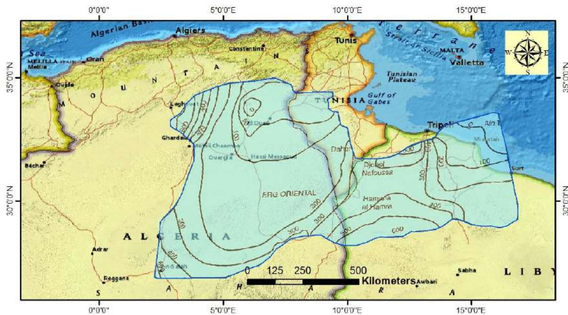
Figure 35. Limites de l'aquifère du Complexe Terminal (OSS, 2003b). Modifier
