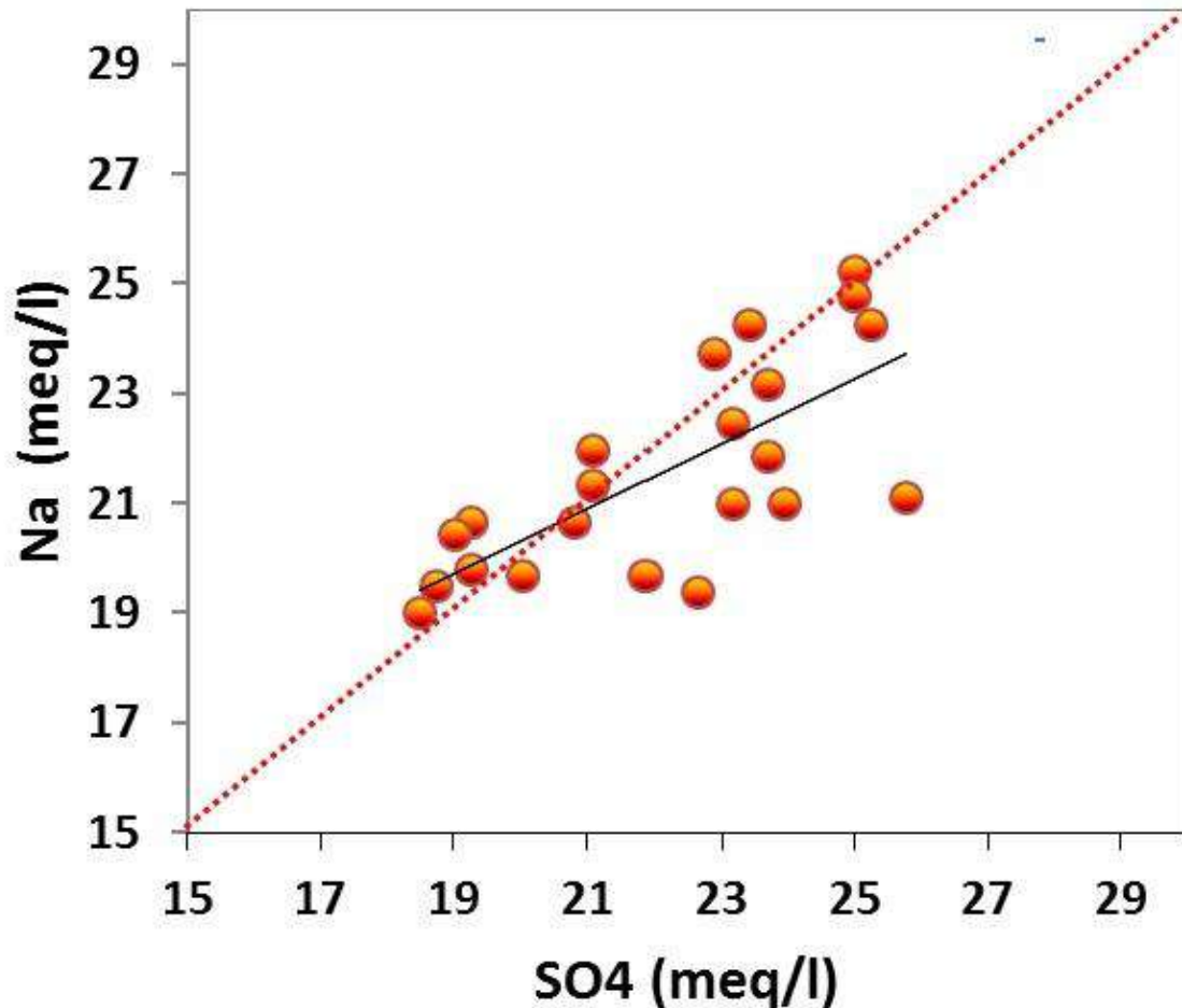
Figure 72: Relation entre \text{Na}^+ et \text{SO}_4^{2-}
