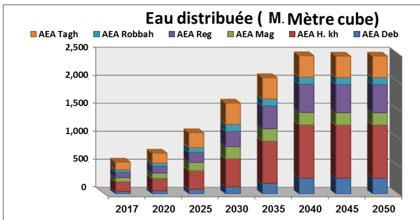
Figure 103. L'eau distribuée - Scénario 1 : Scénario de référence (2018-2050)-
