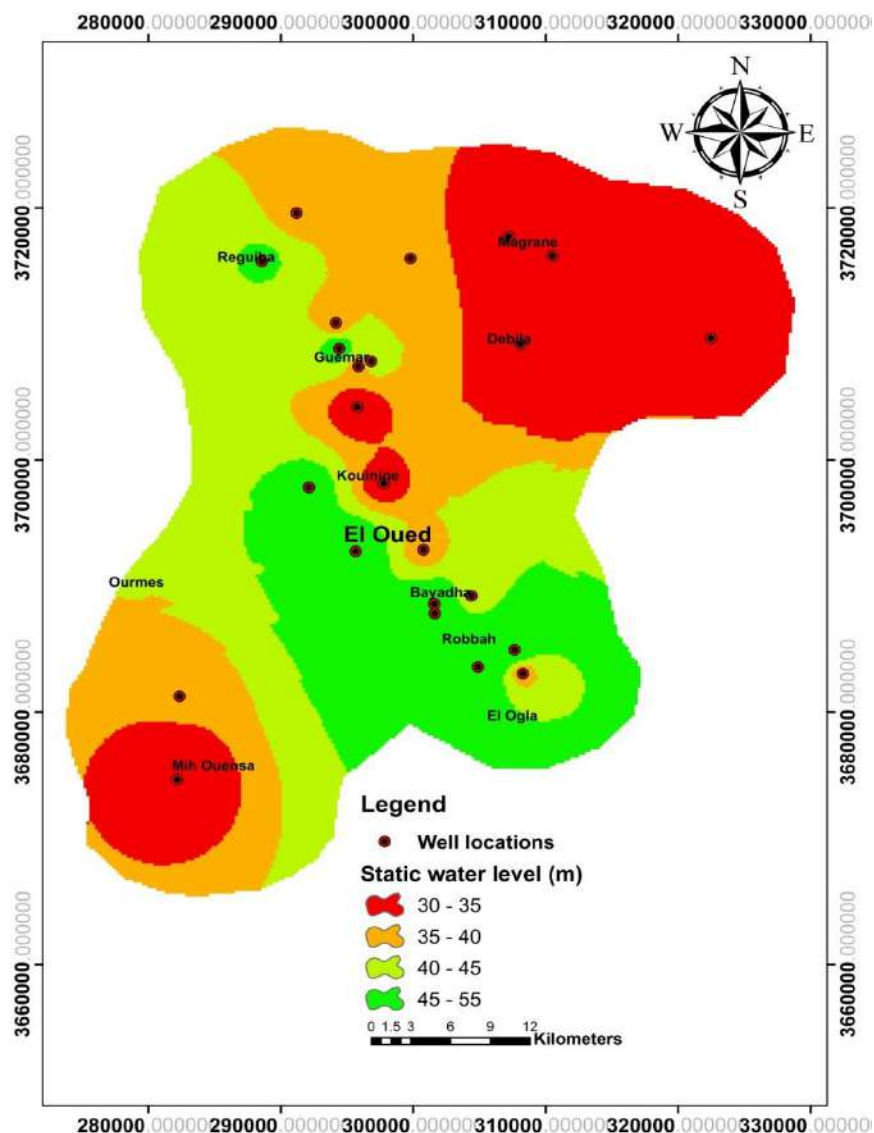
Figure 51: Distribution spatiale de niveau statique de l'aquifère CT.
