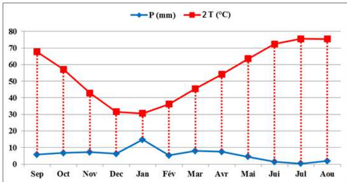
Figure 12: Courbe Pluvio-thermique d'El-Oued (1978-2017)
