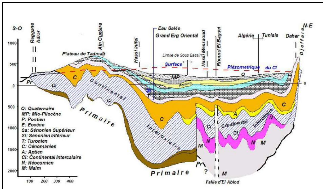
Figure 40 : Coupe hydrogéologique du système aquifère CI et CT (UNESCO, 1972)
