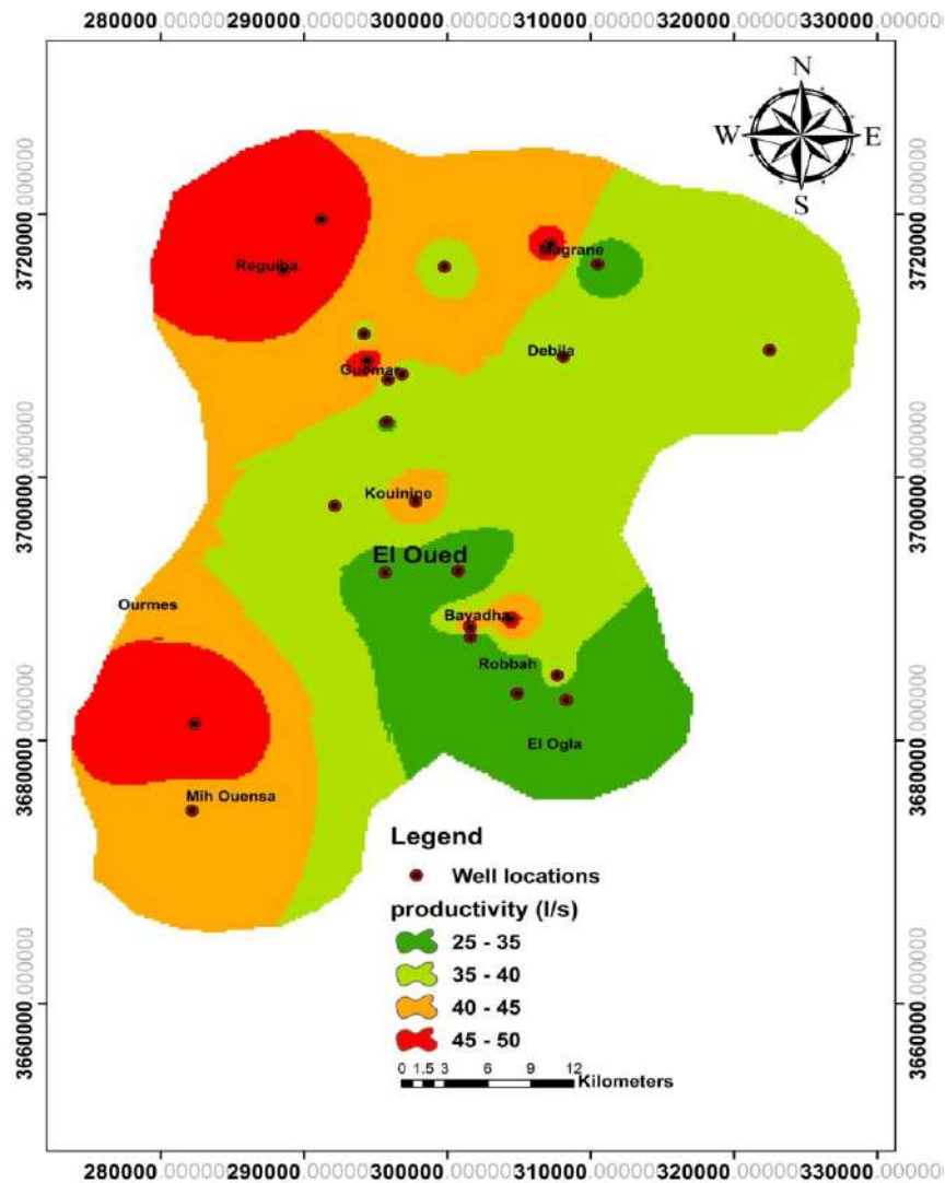
Figure 48: Distribution spatiale de la productivité de l'aquifère CT.
