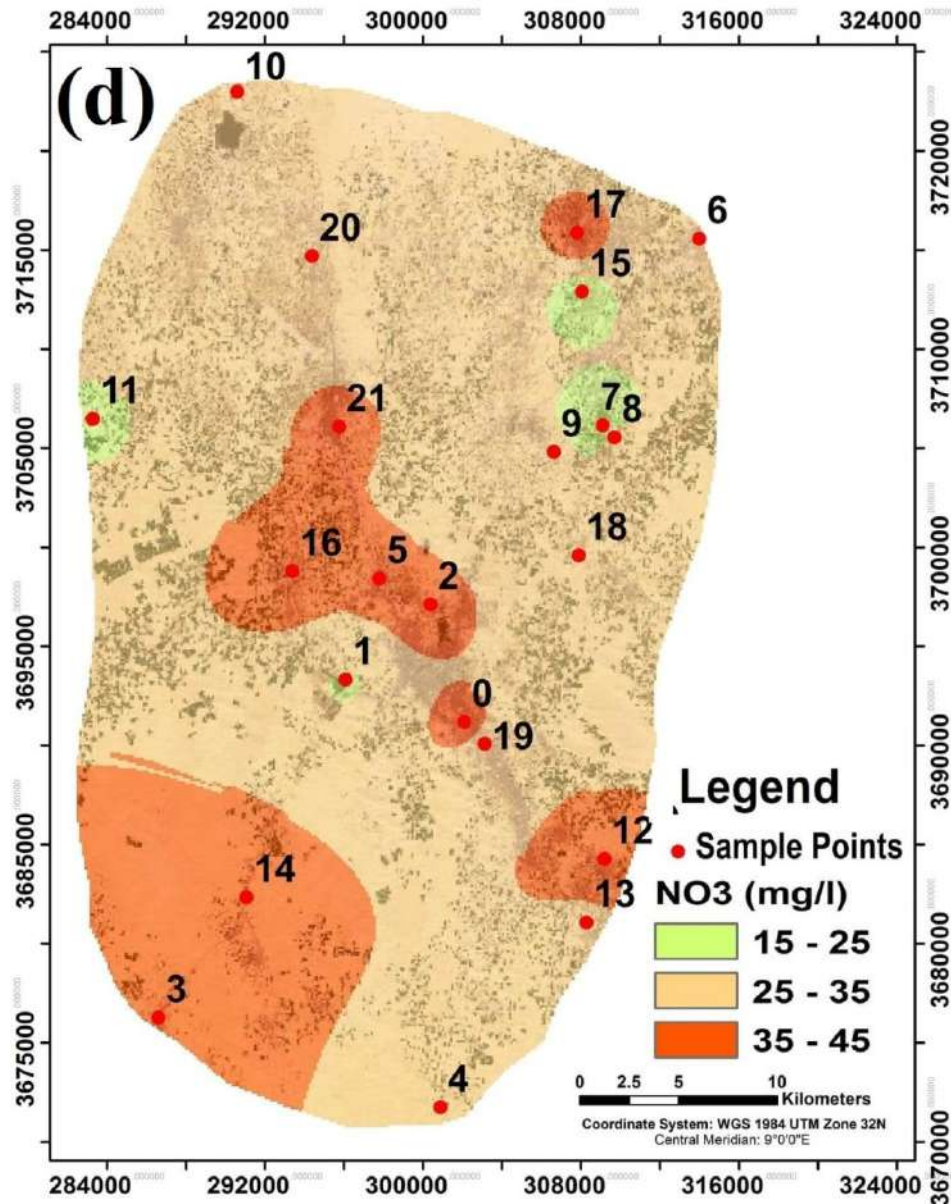
Figure 64: Carte de distribution spatiale des nitrates
