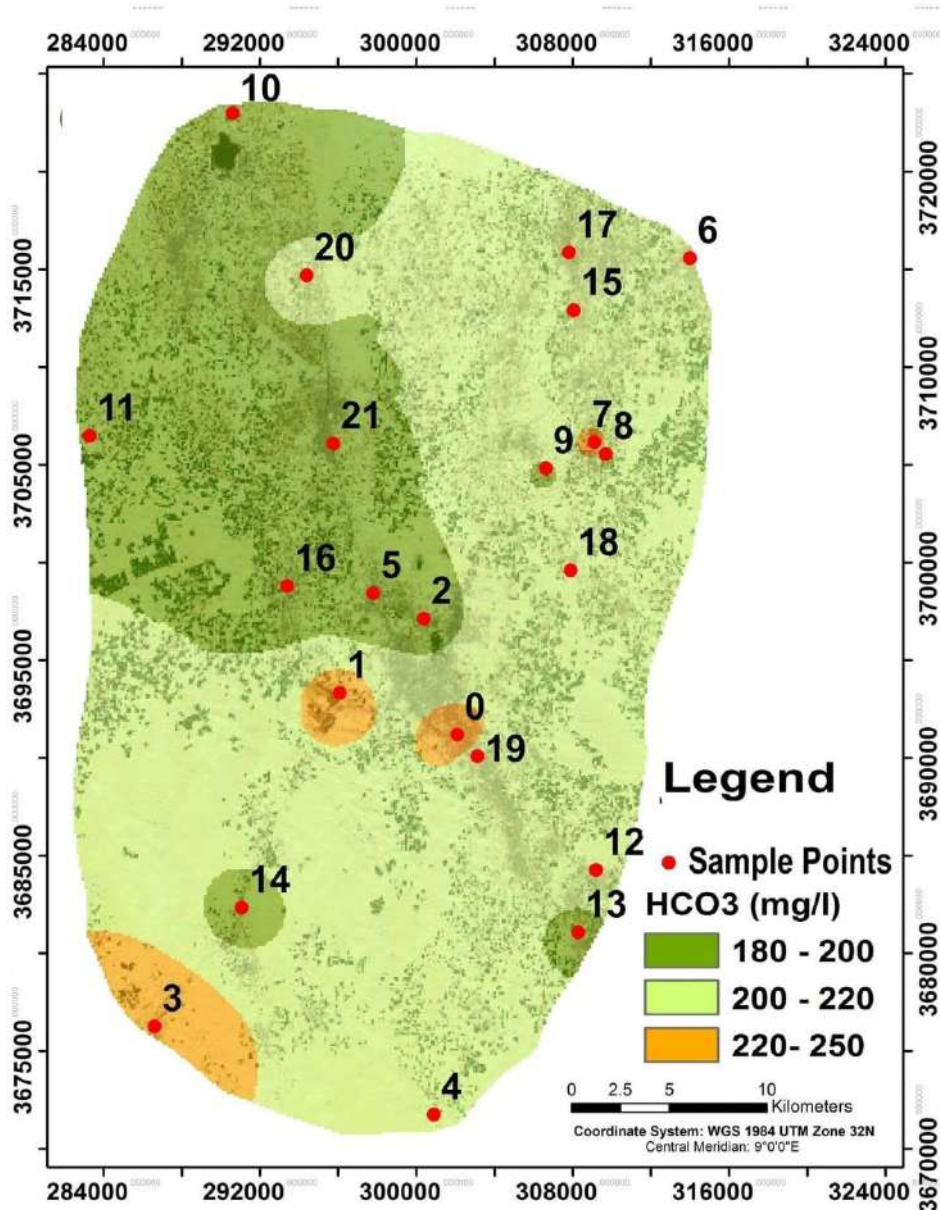
Figure 63: Carte de distribution spatiale des bicarbonates
