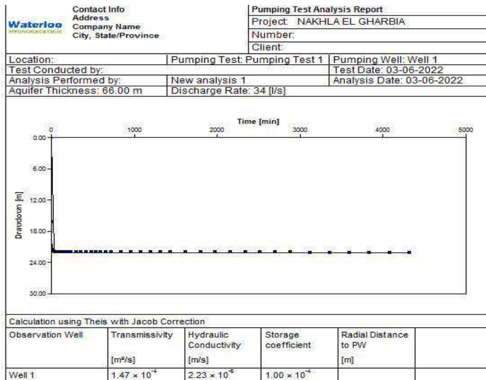
Figure 45. Essai de pompage longue durée à Nakhla
