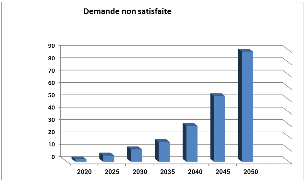
Figure 108. Demande en eau non satisfaite. - Scénario 2 : Fort accroissement de la population (2018-2050)-
