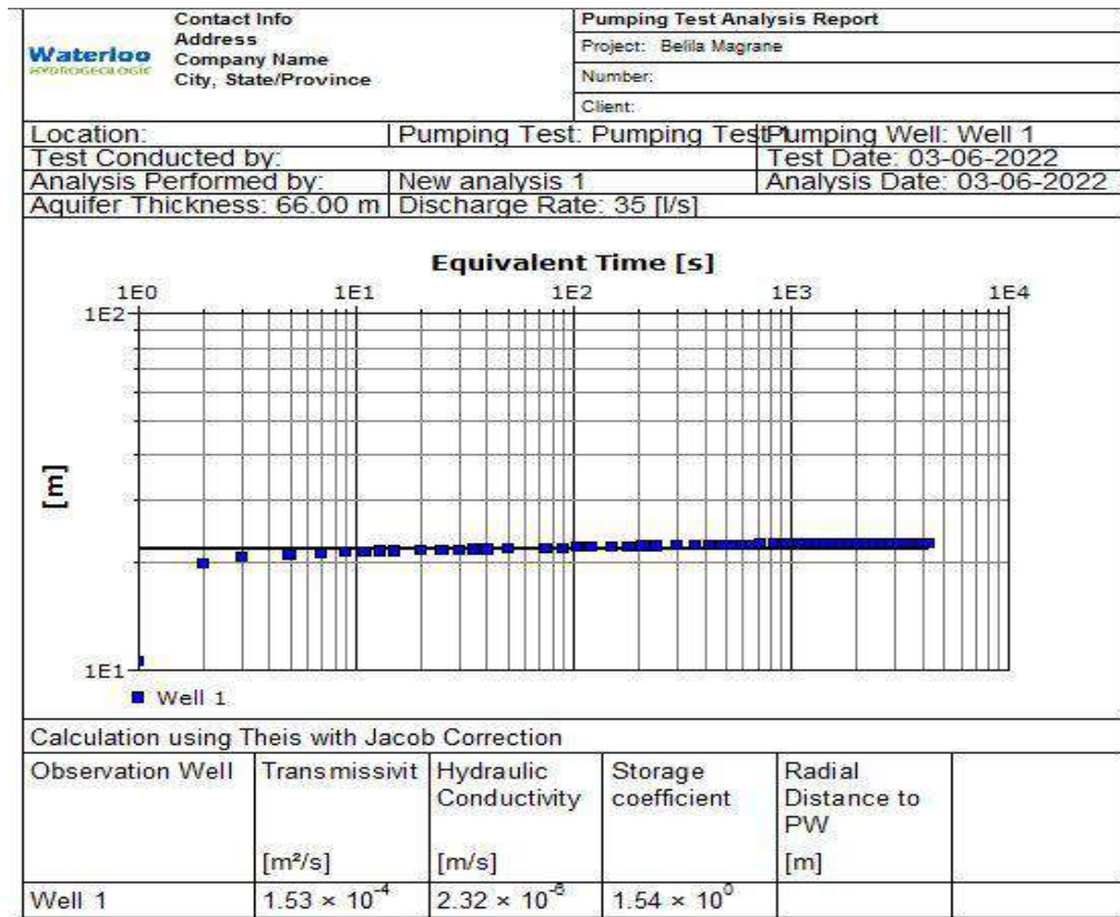
Figure 46: Essai de pompage longue durée à el Magrane
