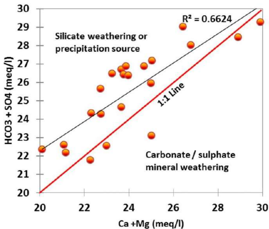
Figure 74: Diagramme de (\text{Ca}^{2+}+\text{Mg}^{2+}) en fonction de (\text{HCO}_3 + \text{SO}_4^{2-}) en meq/l.
