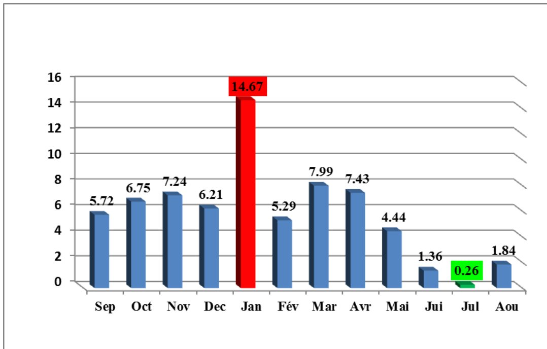
Figure 10: Histogramme des précipitations moyennes mensuelles (1978-2017).
