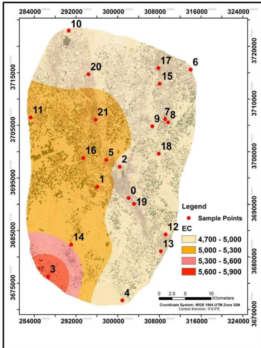
Figure 56: Carte de distribution spatiale de la conductivité électrique
