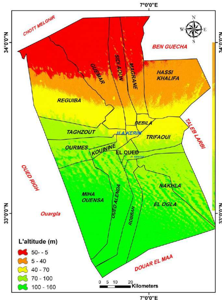
Figure 04 : Topographie de la zone d'étude
