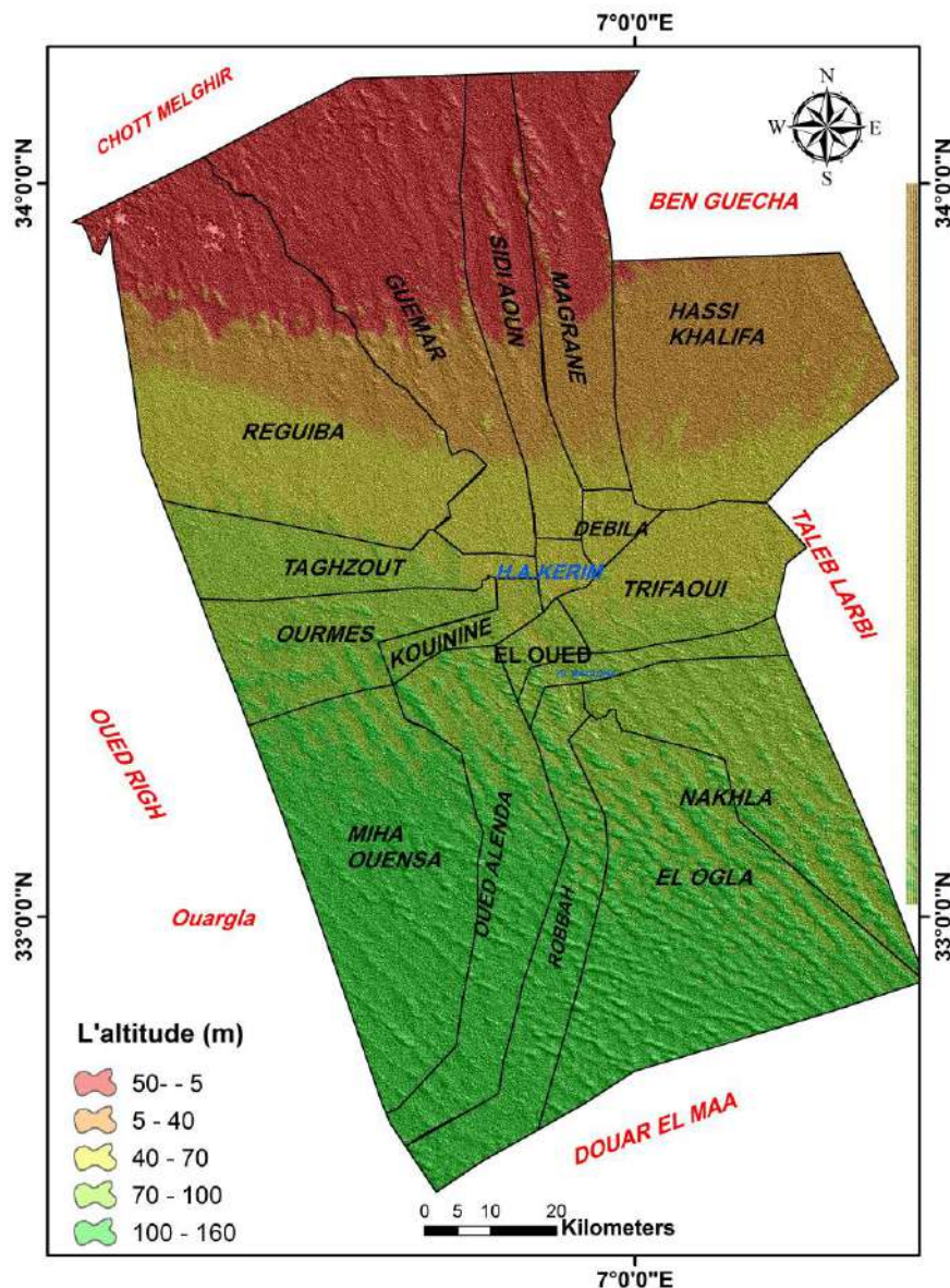
Figure 05 : Géomorphologie de la région d'étude
