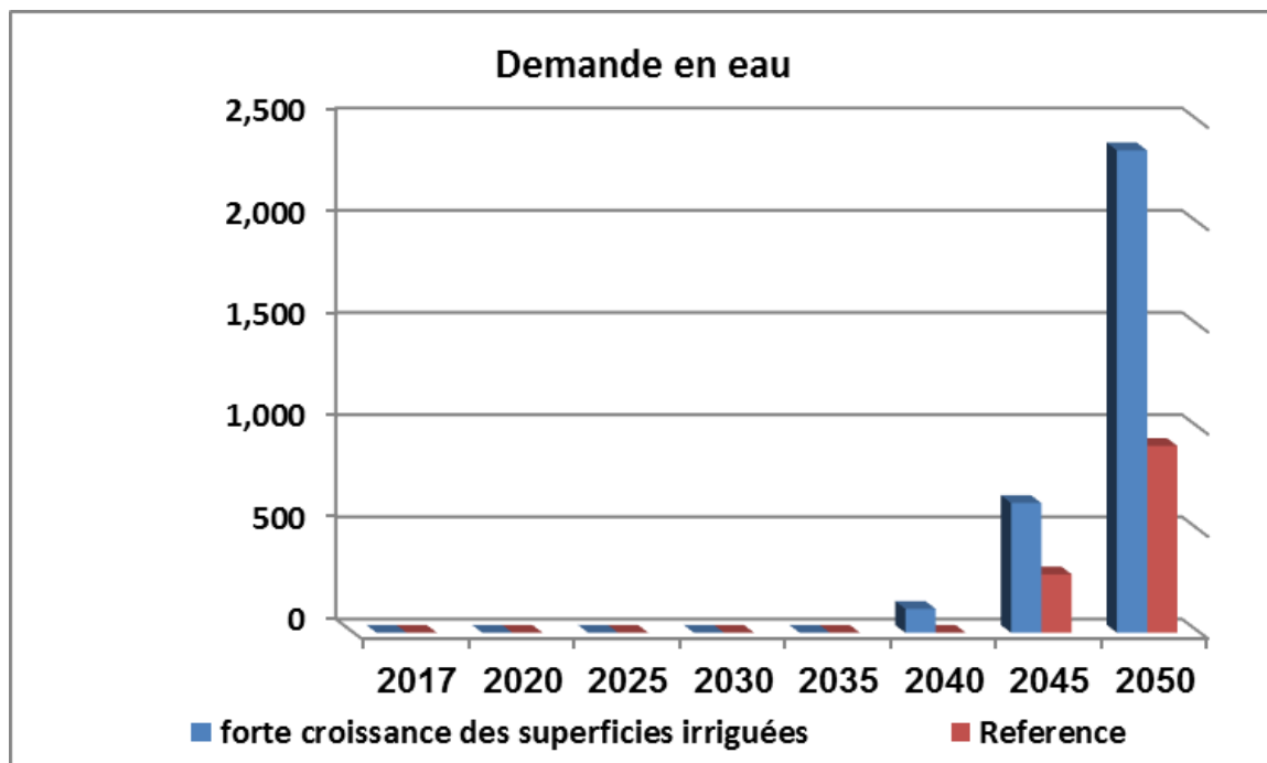
Figure 117. Evolution de la demande non satisfaite - Comparaison avec le scénarios (2018-2050)-
