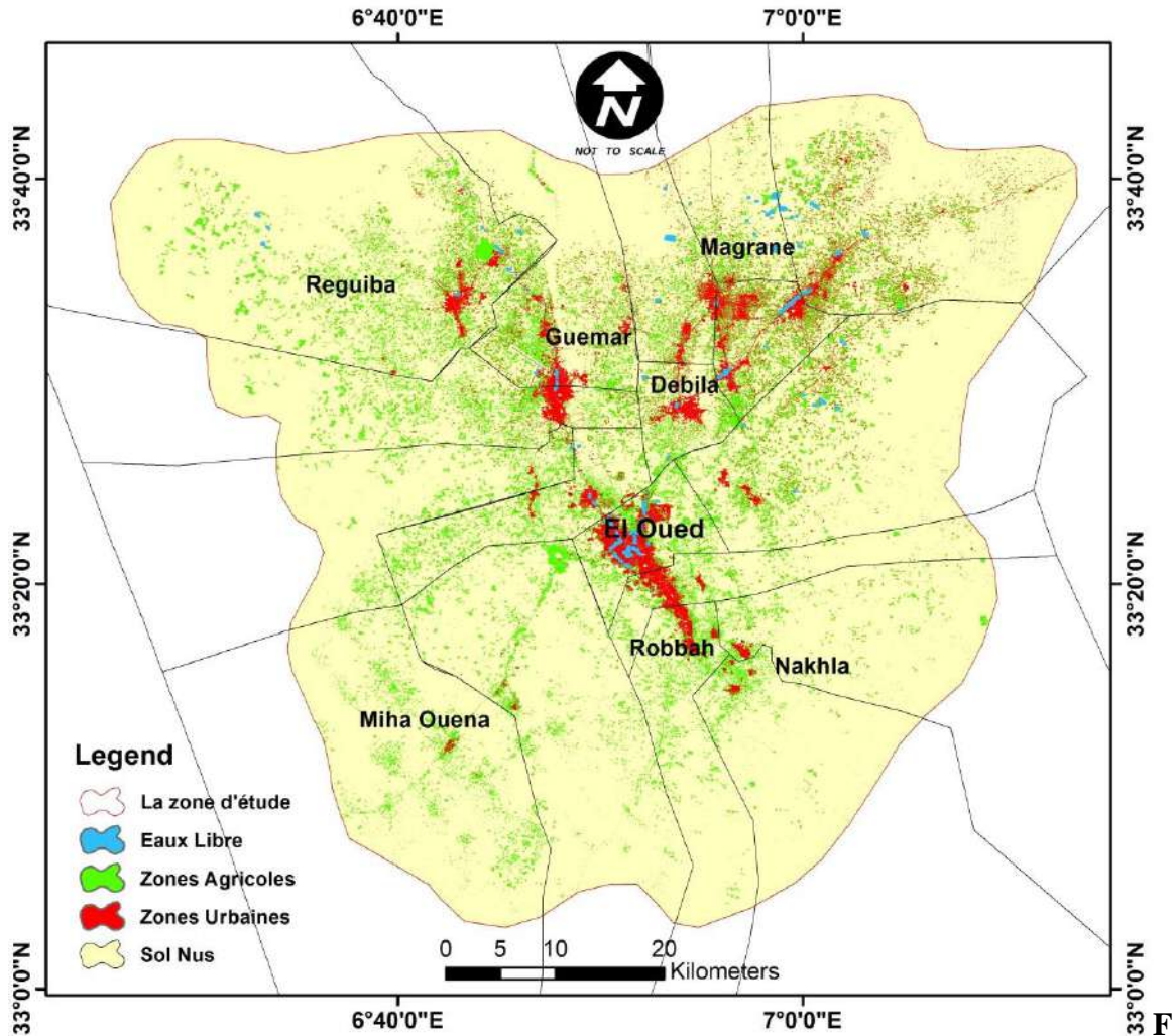
Figure 08: carte d'occupation de sol de région d'étude (2020)
