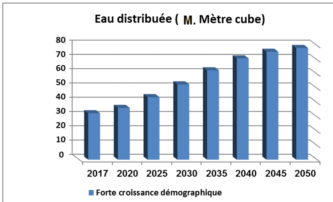
Figure 107. Eau distribuée. -Scénario 2 : Fort accroissement de la populaion (2018-2050)
