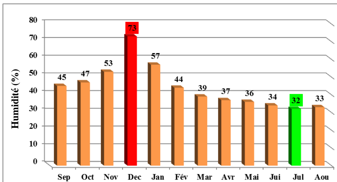
Figure 14 : Histogramme d'humidité relative moyenne mensuelle (1997 – 2017)
