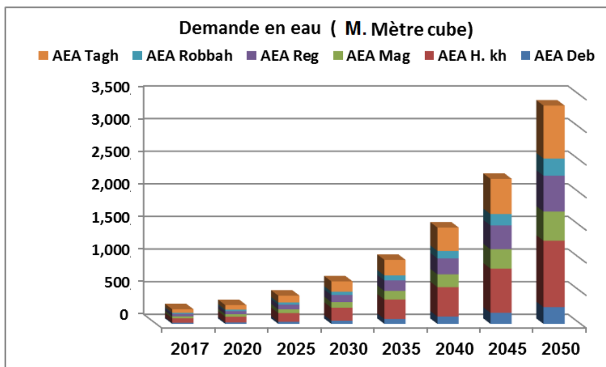
Figure 102. Demande en eau eau d'irrigation - Scénario 1 : Scénario de référence (2018-2050)-
