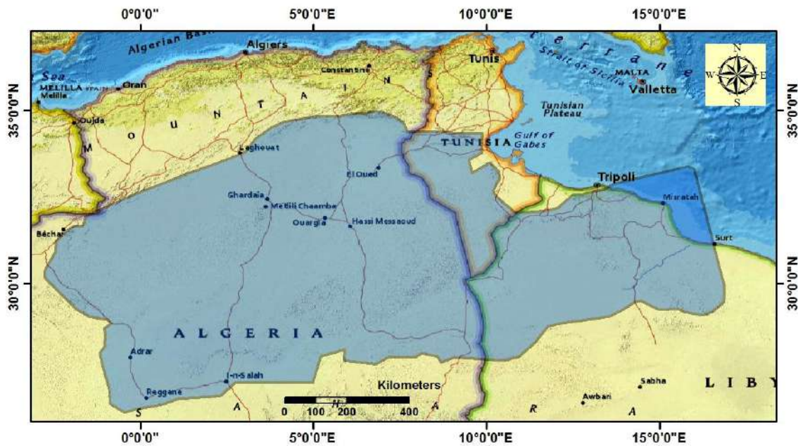
Figure 26 : Limites du Bassin de Système Aquifère du Sahara Septentrional SASS (OSS, 2003) Modifier.
