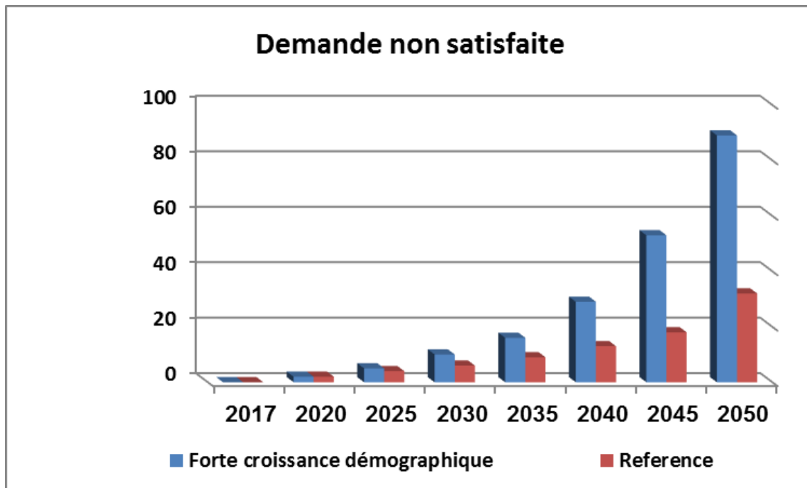
Figure 110. Comparaison de demande non satisfaite avec le scénario référence (2018-2050)-
