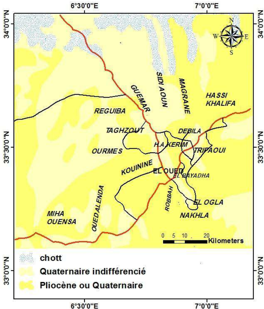
Figure 20 : Carte géologique locale
