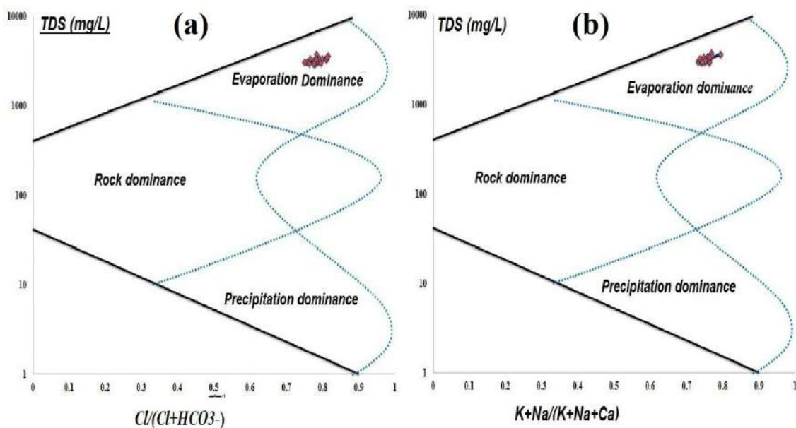
Figure 68: Le plot de l'échantillon d'eau souterraine dans le diagramme de Gibbs
