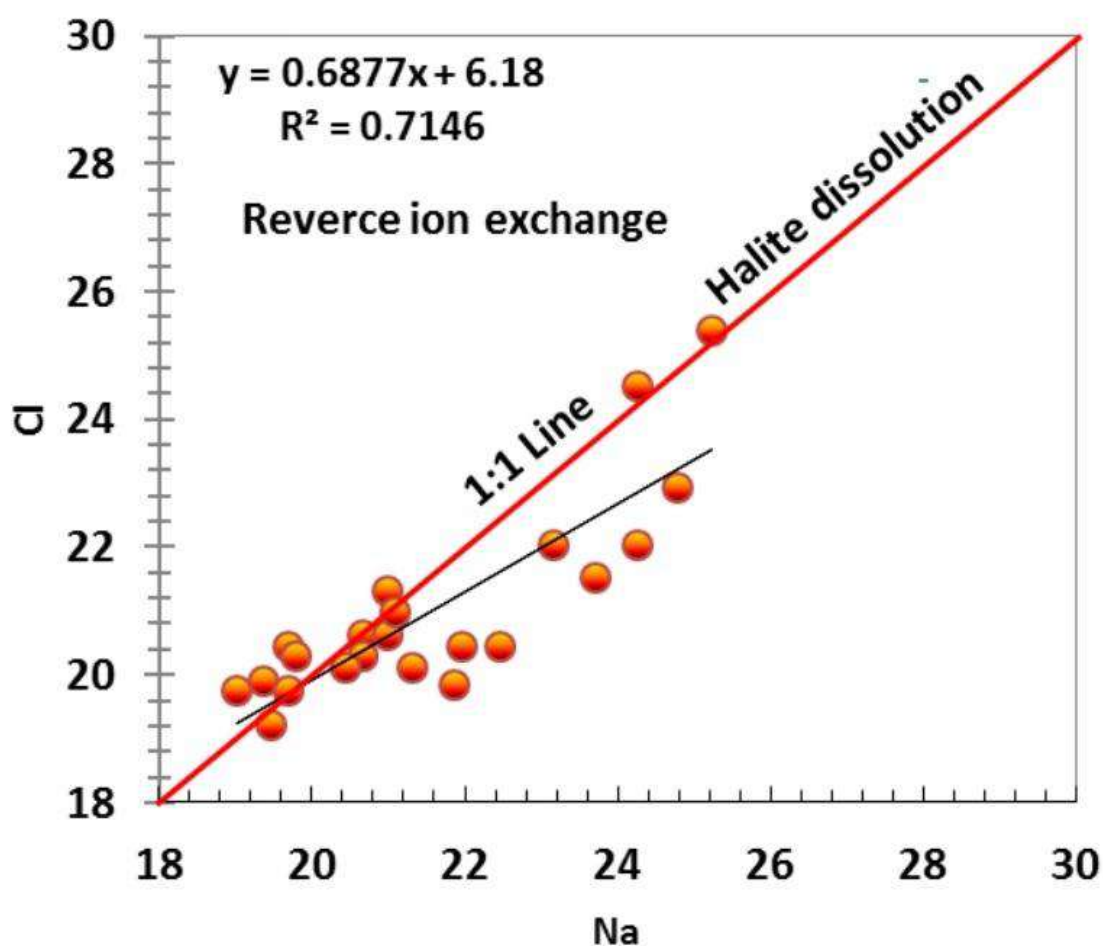
Figure 69: Relation entre \text{Na}^+ et \text{Cl}^-
