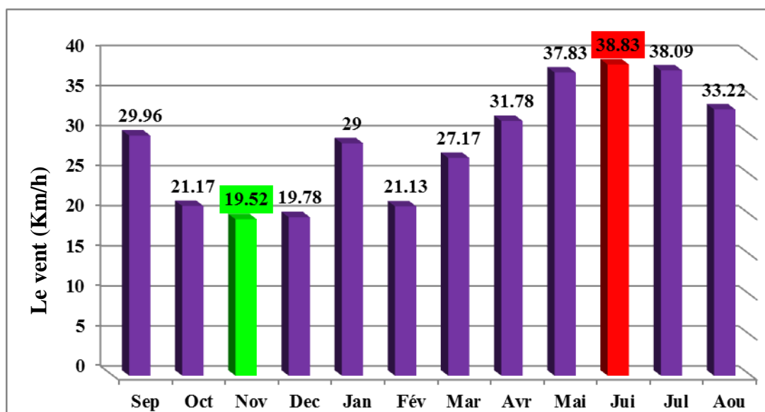
Figure 15 : Histogramme de La vitesse du vent moyenne mensuelle (1997 – 2017)
