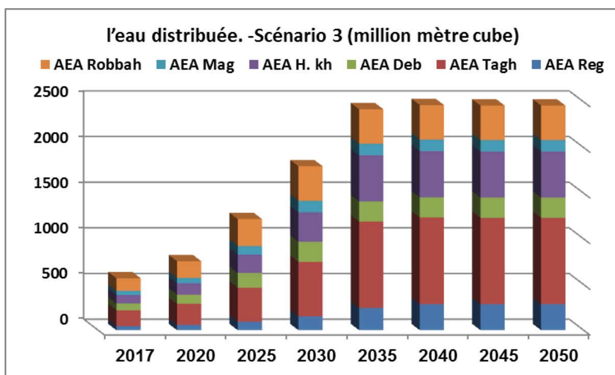
Figure 113. Eau distribuée. -Scénario 3 : Augmentation des superficies irriguées (2018-2050)-
