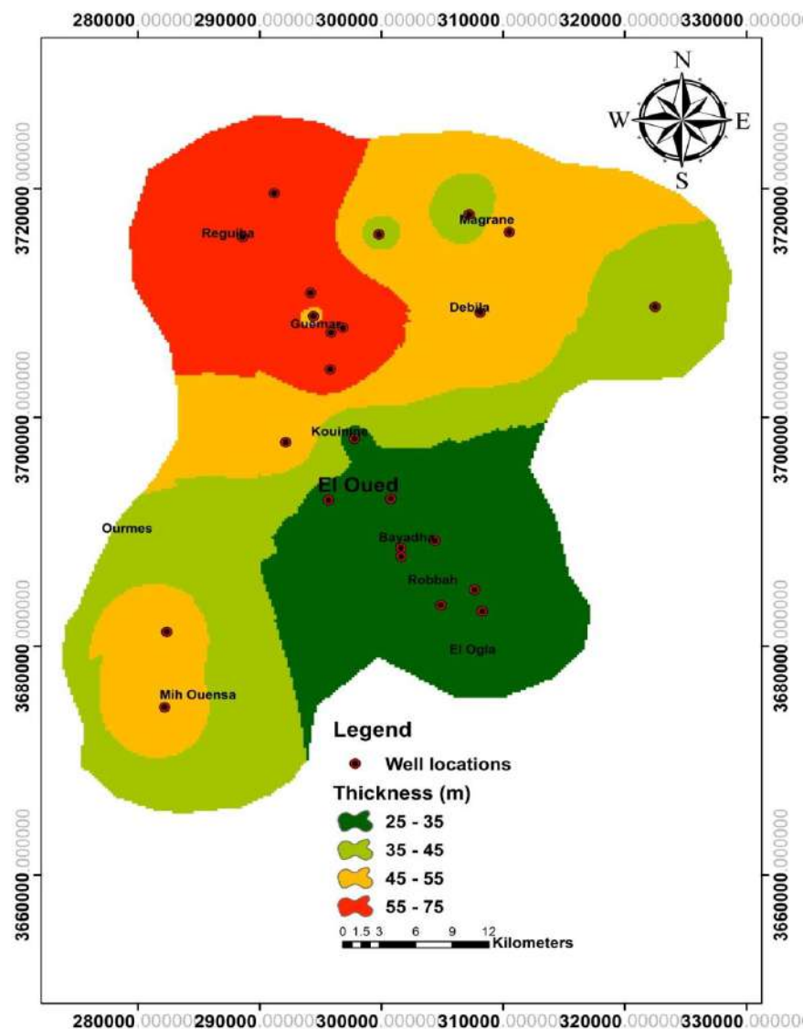
Figure 50: Distribution spatiale de l'épaisseur de l'aquifère CT.
