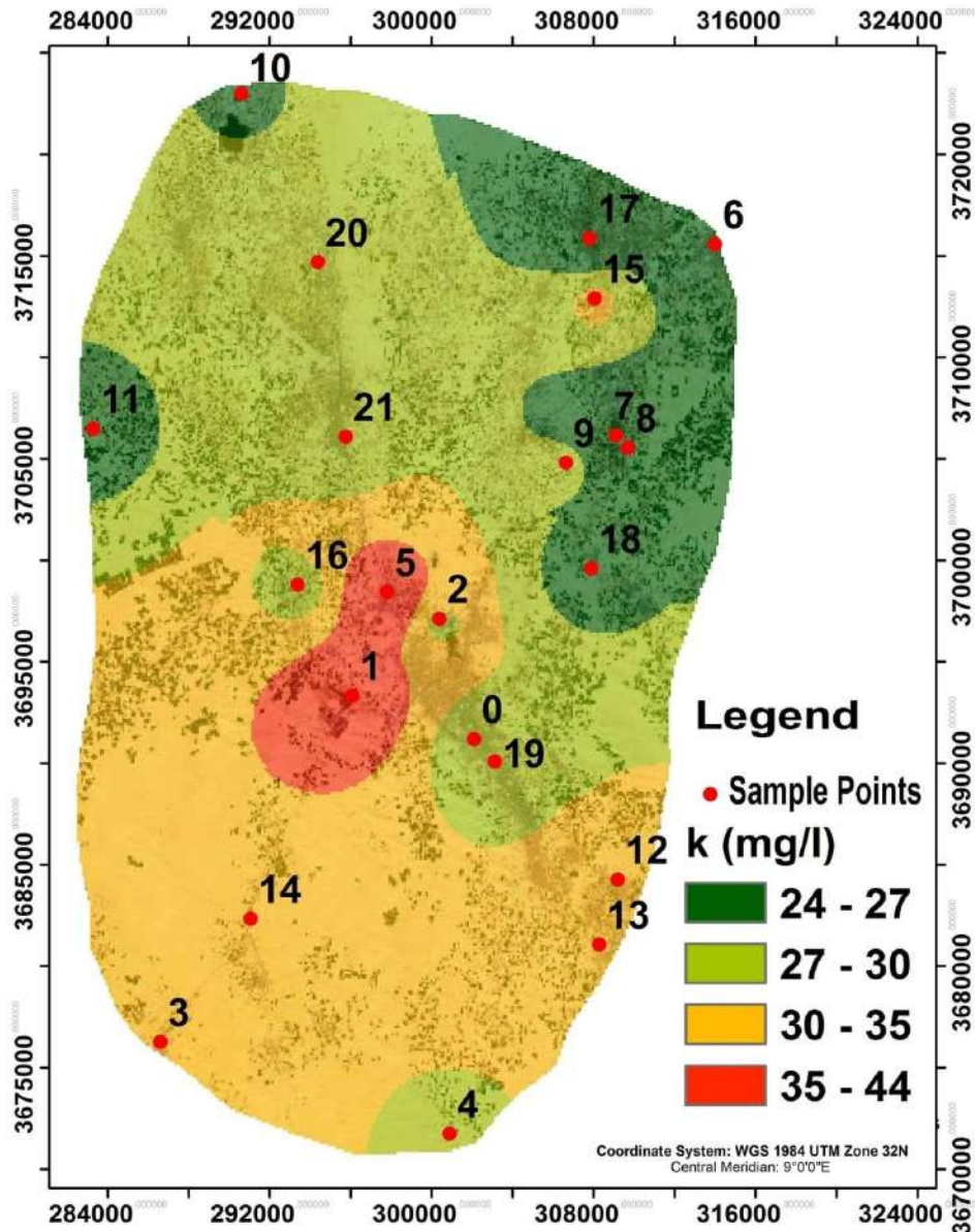
Figure 59: Carte de distribution spatiale de potassium
