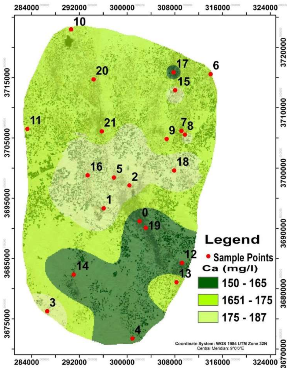
Figure 57: Carte de distribution spatiale de calcium
