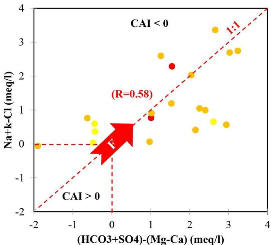
Figure 84: Diagramme de [(Na^{++}K^+) - Cl^-] vs [(SO_4^{2-} + HCO_3^-) - (Ca^{2++}Mg^{2+})] en meq
