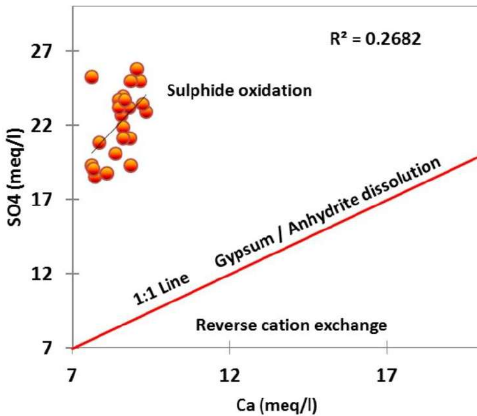
Figure 71: Relation entre a \text{Ca}^{2+} et \text{SO}_4^{2-}
