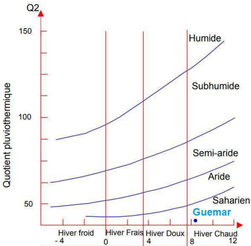
Figure 13: Diagramme d'Emberger de la station d'El-Oued (1978-2017)
