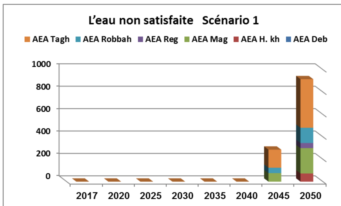
Figure 104. Demande en eau non satisfaite - Scénario 1 : Scénario de référence (2018-2050)-
