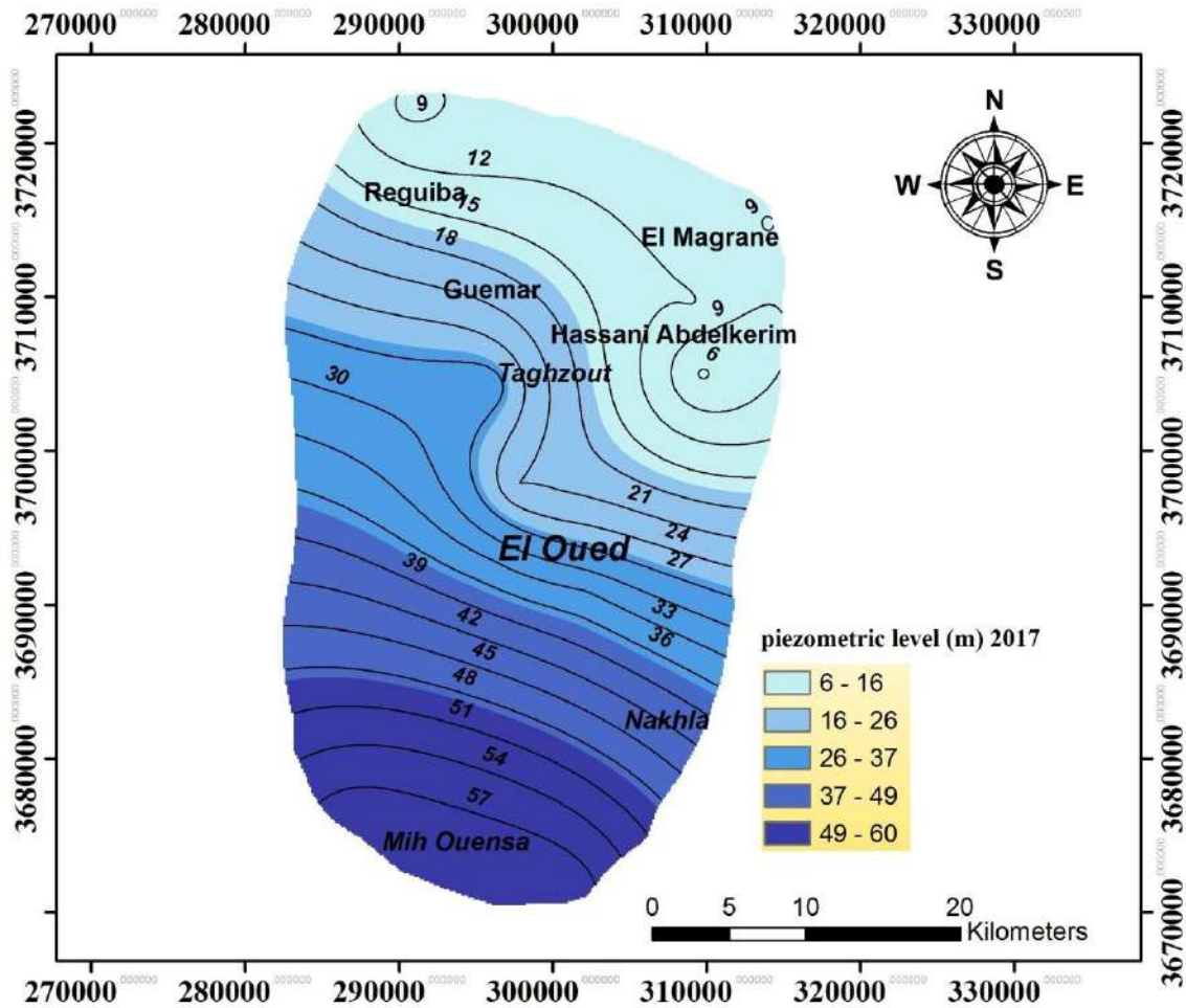
Figure 37: Carte du niveau piézométrique des eaux souterraines des aquifères du CT (mars 2017).
