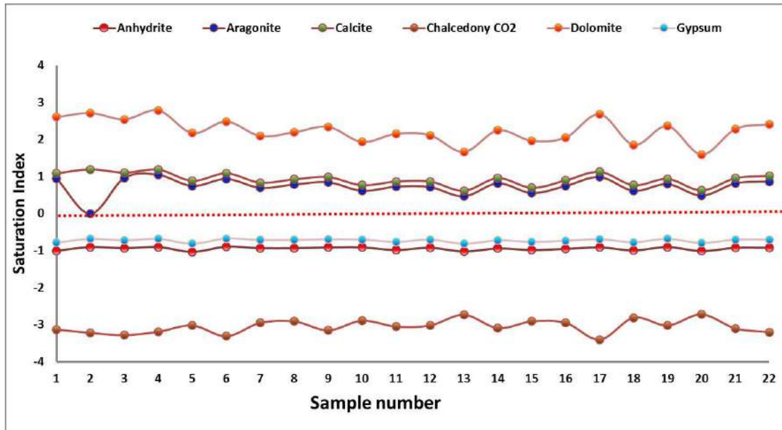
Figure 75: Diagramme de l'état de saturation de minéral de l'aquifère CT
