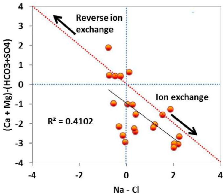
Figure 73: Diagramme de [(\text{Na}^++\text{K}^++\text{Cl}^-)] en fonction de [(\text{Ca}^{2+}+\text{Mg}^{2+})-(\text{SO}_4^{2-} + \text{HCO}_3^-)] en meq/l
