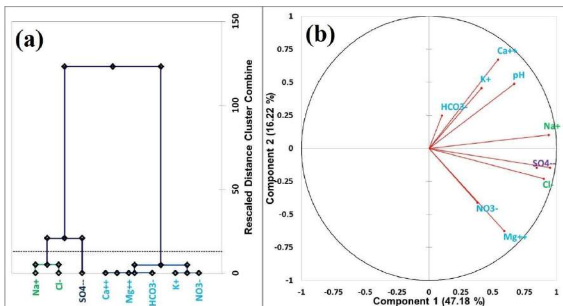
Figure 76: Dendrogramme HCA des paramètres des eaux souterraines (a), résultats de l'ACP montrant les variables des PC1 (b)
