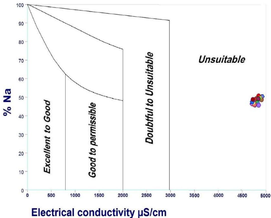
Figure 66: Représentation graphique de la classification de l'eau pour usage d'irrigation,
