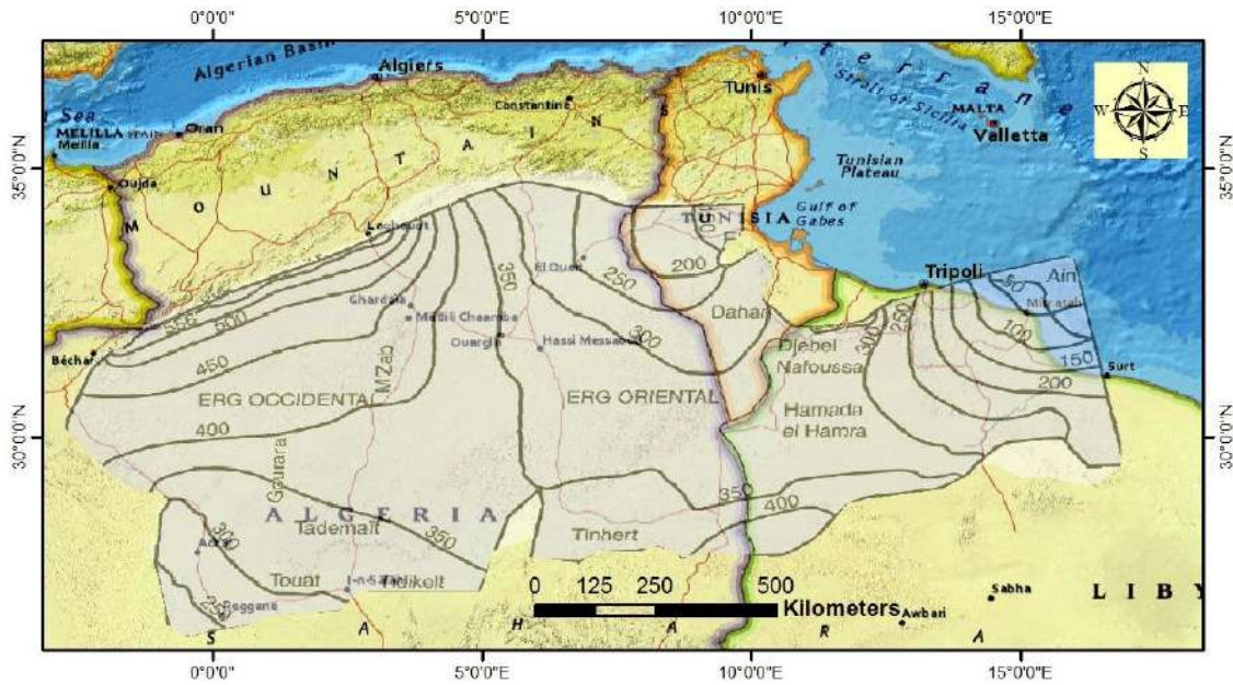
Figure 41: Limite et piézométrie du Continental Intercalaire (Baba SY et al., 2006).
