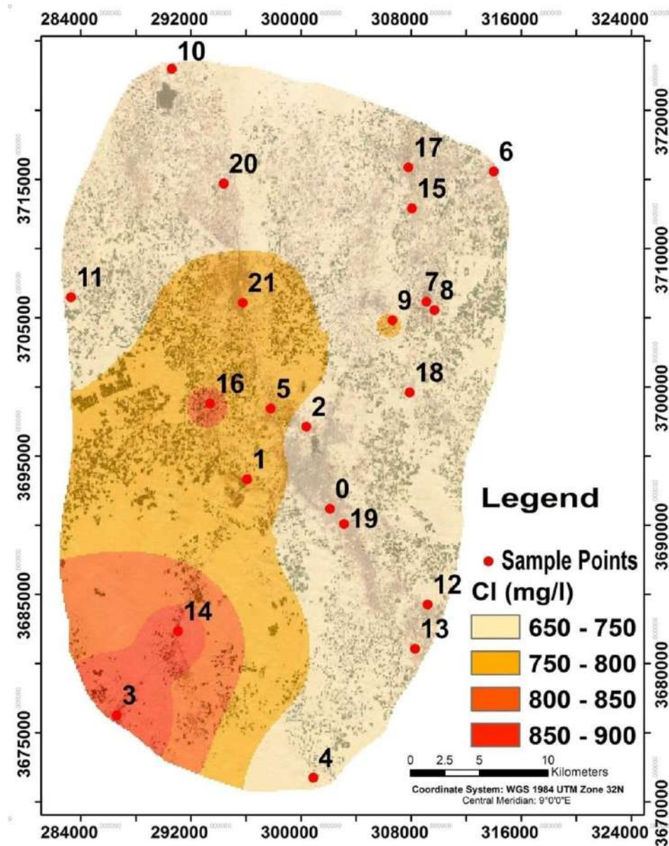
Figure 62: Carte de distribution spatiale des chlorures
