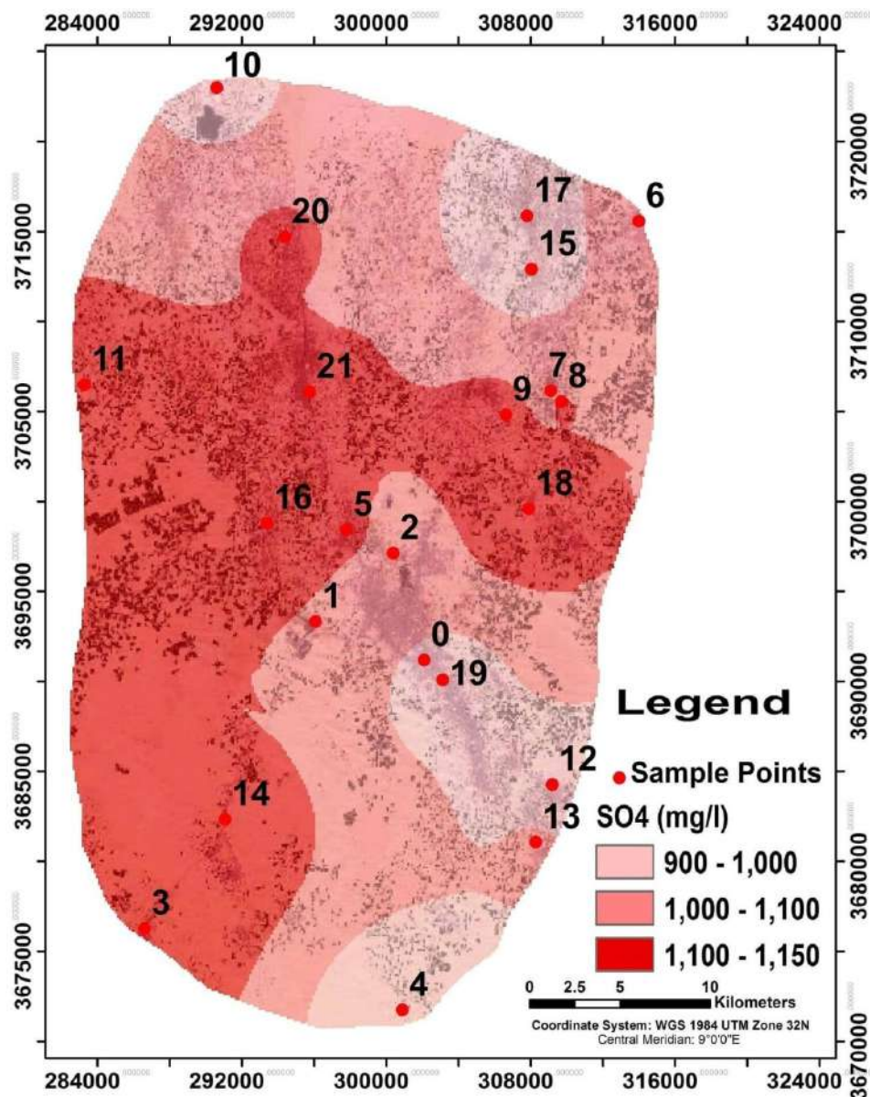
Figure 61: Carte de distribution spatiale de sulfates
