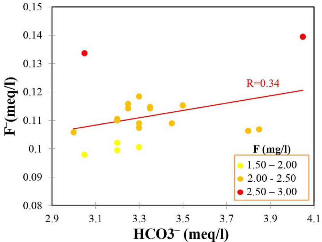
Figure 82: Relation entre F - et HCO 3 -
