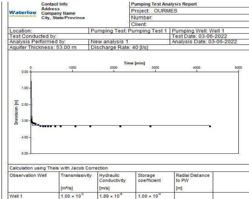
Figure 44: Essai de pompage longue durée à Ourmes
