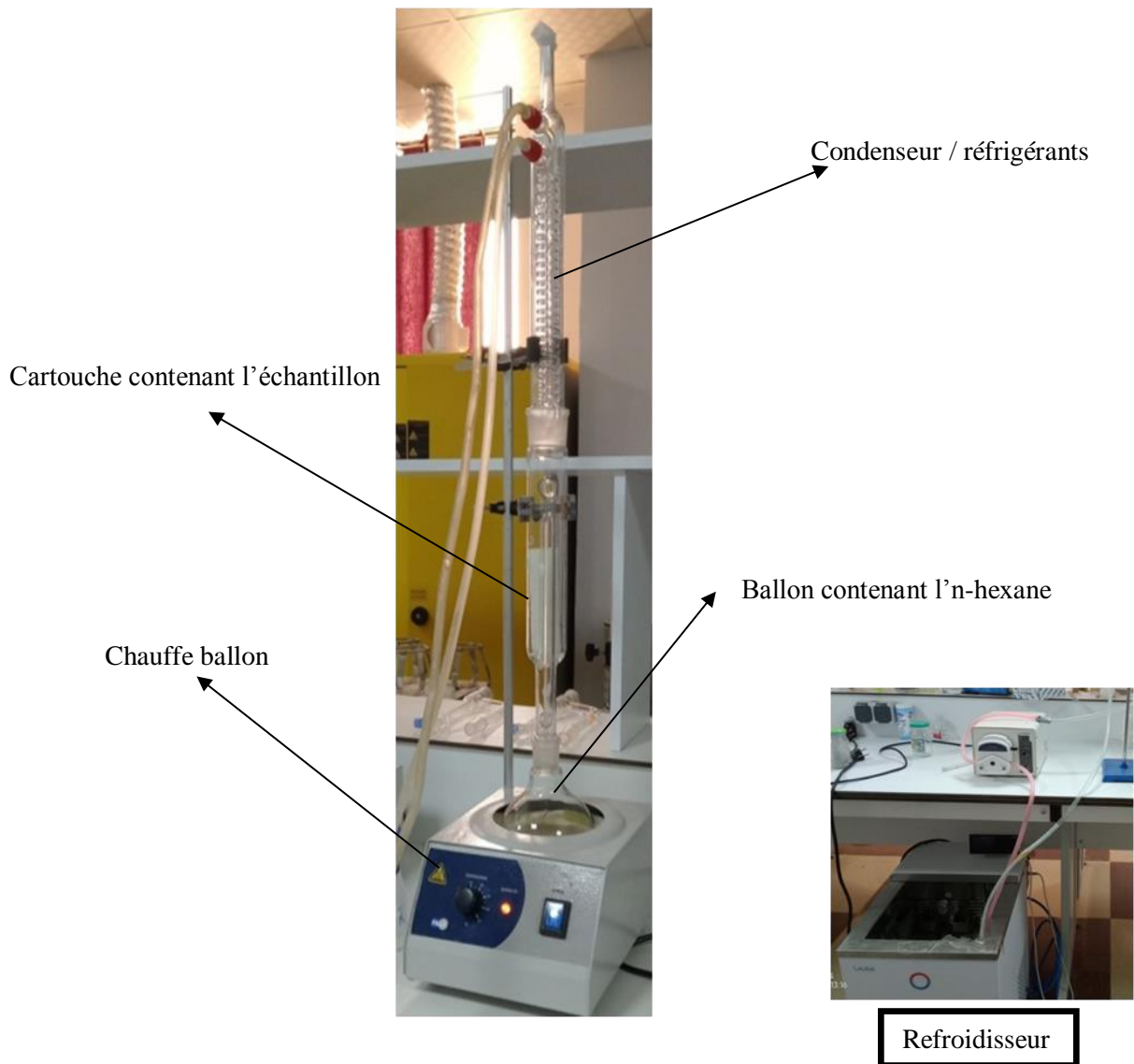
Figure N°21. Dispositif du soxhlet.
