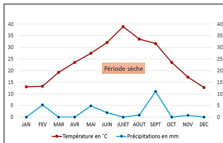
Figure N° 2 : Diagramme ombrothermique de la région d'Ouargla (2008 - 2018)
