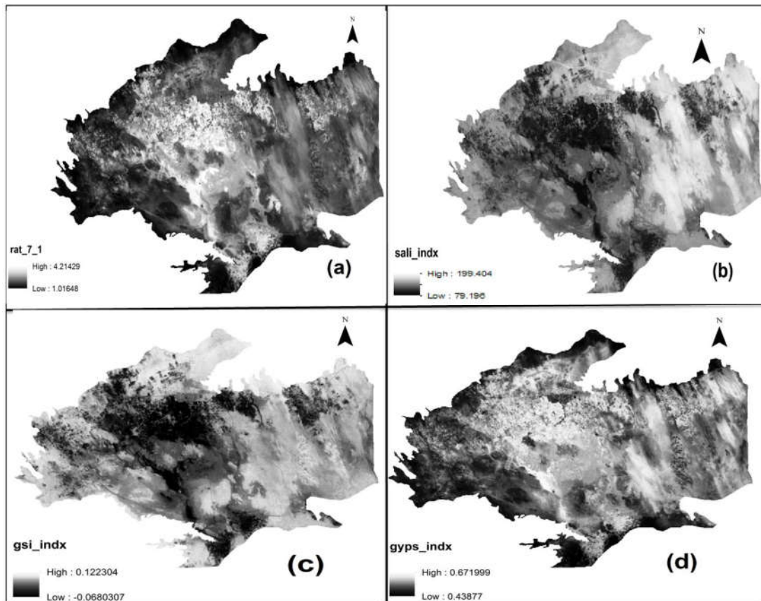
Figure 6. Les indices spectraux calculés à partir de l'imagerie Landsat 5 TM. rat_7_1(a), sali_indx (b), gsi_indx (c) et gyps_indx (d).
