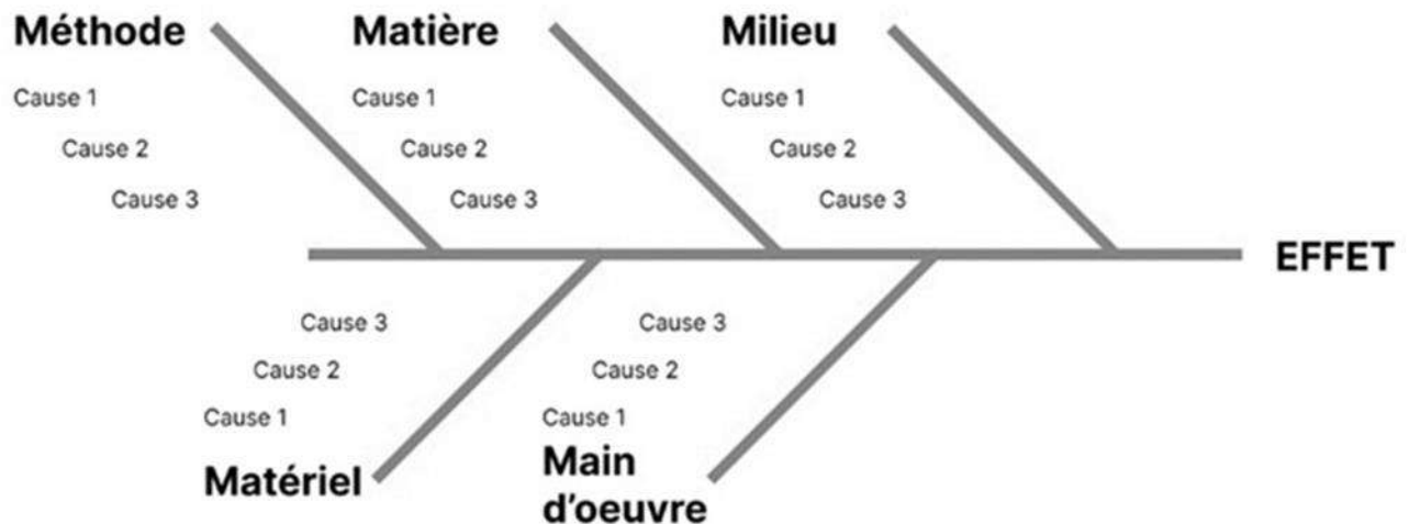
Figure. II.1. Représentation de la méthode des 5M
