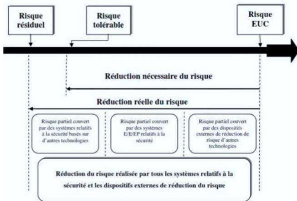
Figure II.4. Reduction du risque : concepts généraux
