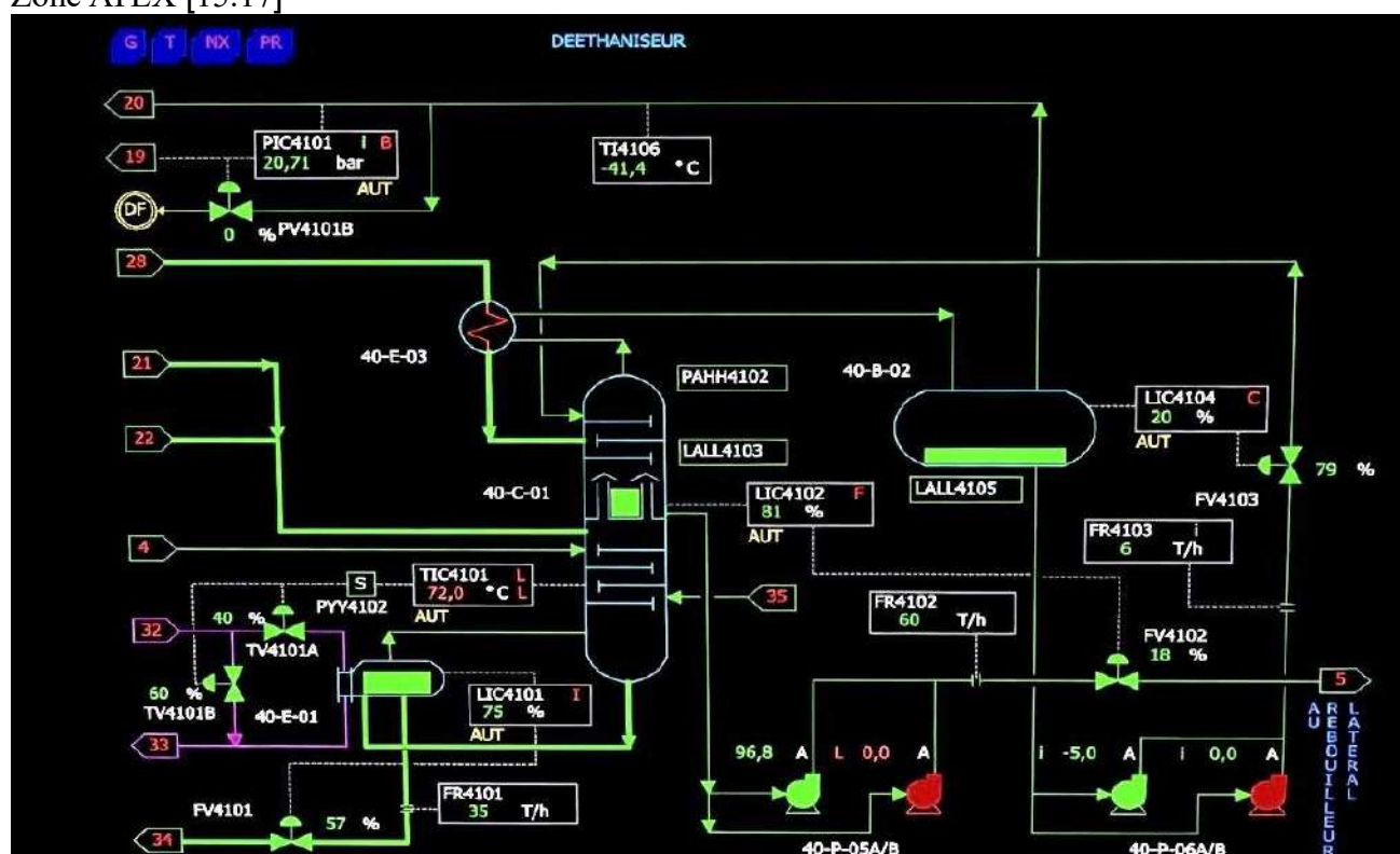
Figure. III.1.PFD Colonne Déméthaniser
