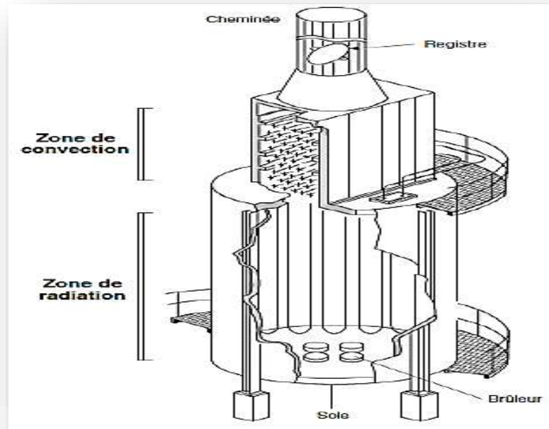
Figure III.1 : Schéma simplifié du Four
