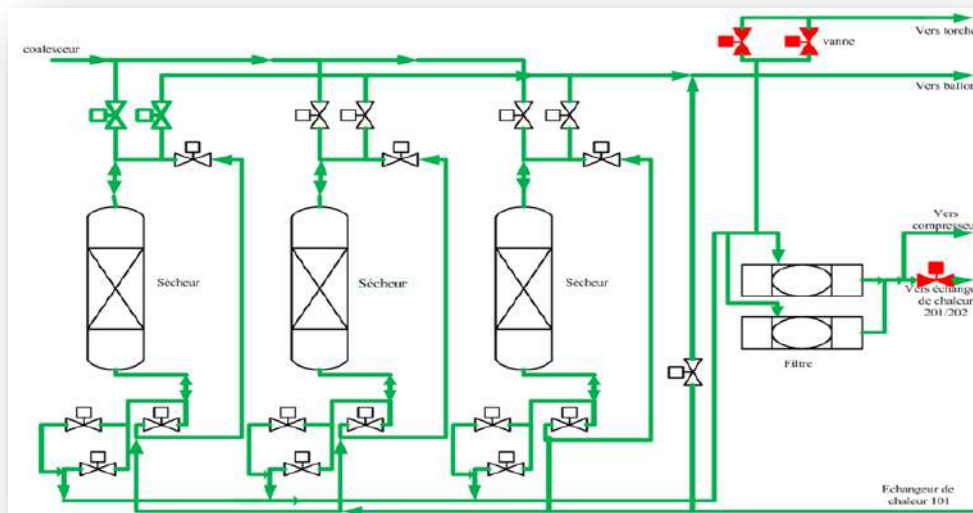
Figure II.4 : Déshydrateurs de gaz (G11).
