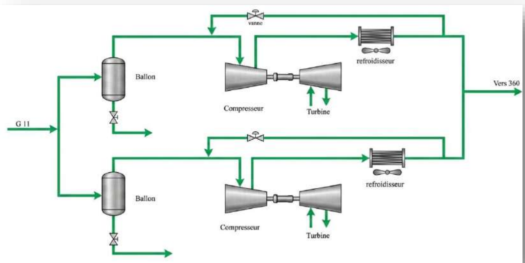
Figure II.8 : Unité de compression de gaz résiduel (G50).
