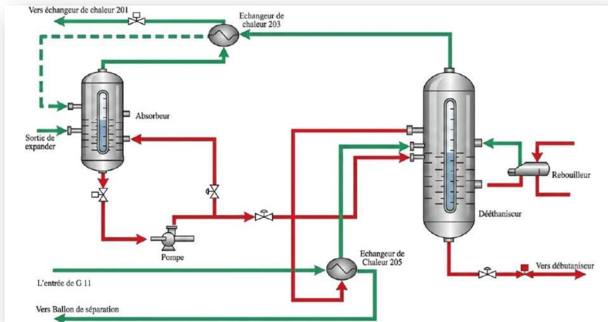
Figure II.7 : Absorbeur/Dééthaniseur (G11).
