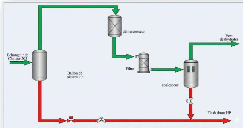
Figure II.3: Séparateur d'entrée, démercuriseur, filtre et coalesceur (G11).
