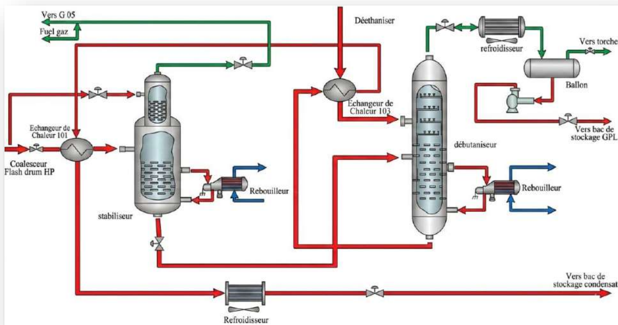
Figure II.9 : Unité de stabilisation de condensât/débutanisations (P10).
