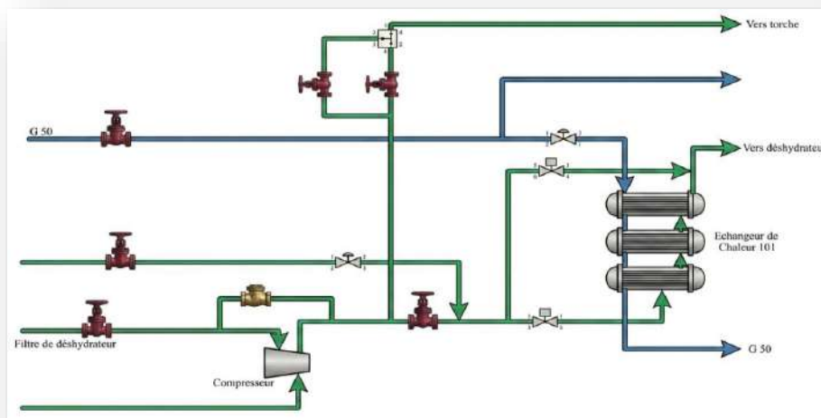
Figure II.5 : Gaz de régénération (G11).
