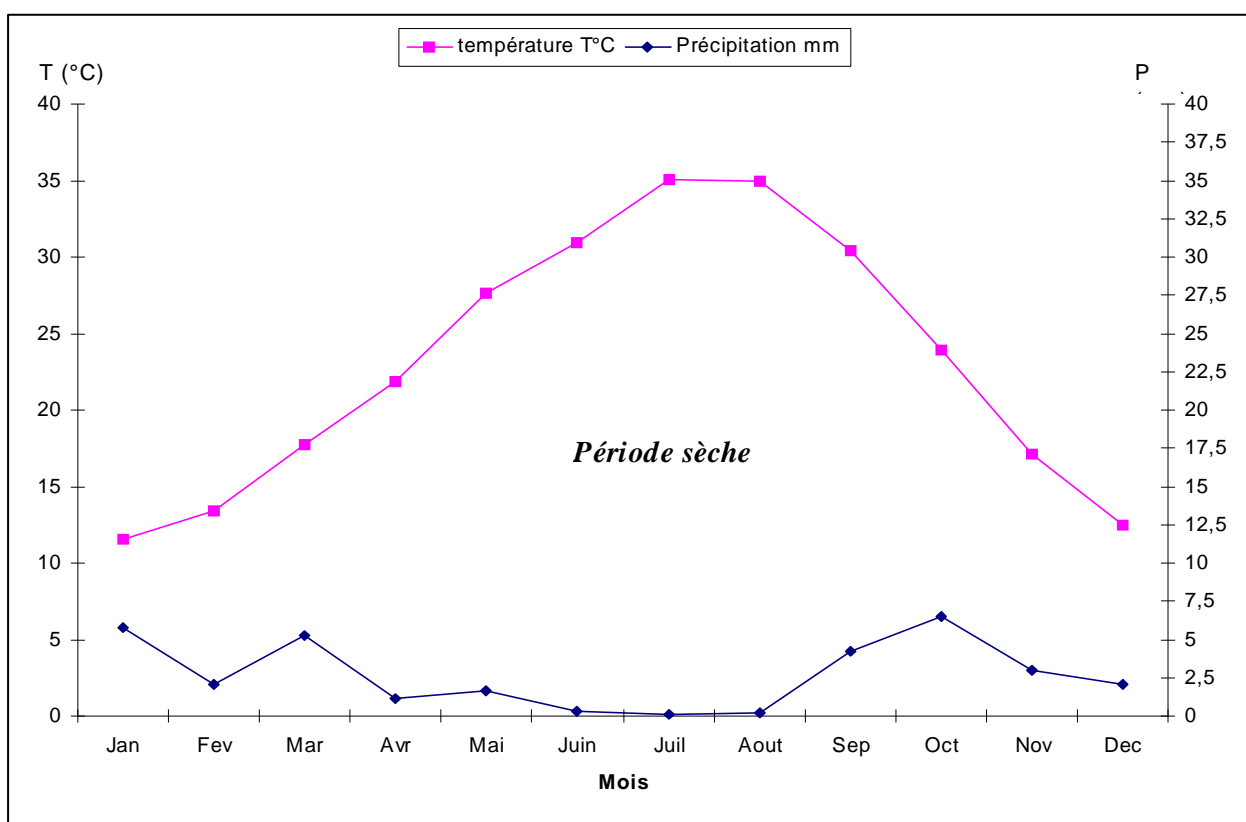
Figure 4 : Diagramme ombrothermique de Ouargla (1993-2003)
