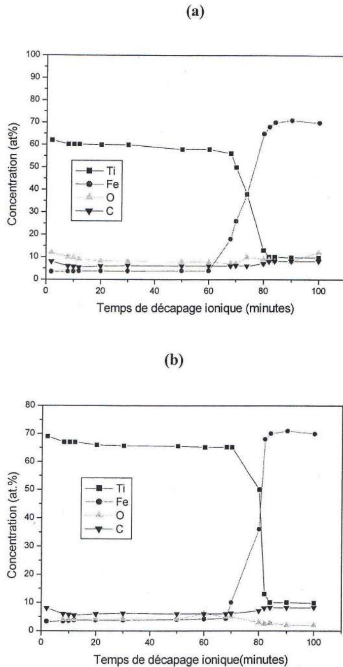
Figure 37: Profils AES de concentration obtenus sur l'échantillon 100C6/Ti, avant recuit : (a) série1, (b) série 2.
