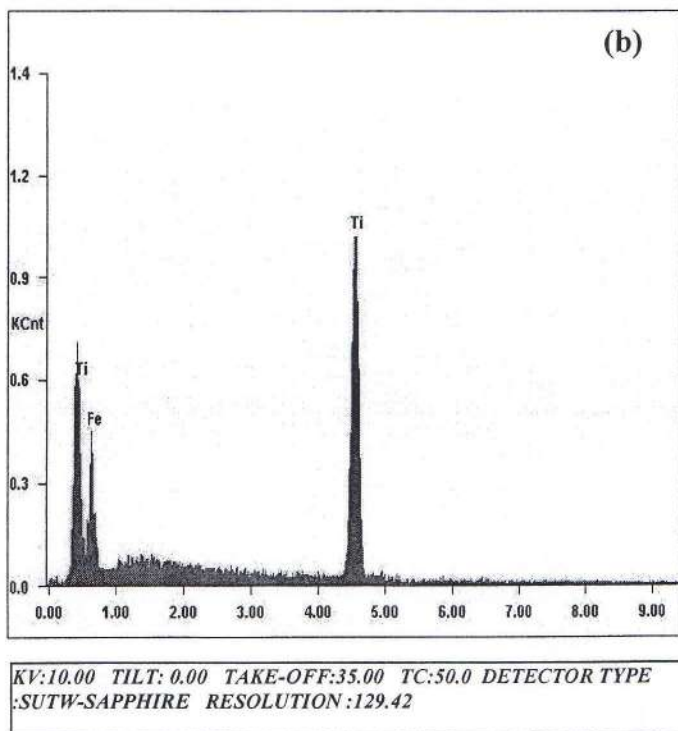
Figure 32: Analyse qualitative et quantitative avec microanalyse x des échantillons : 100C6/Ti, non recuit : (a) série 1 ; (b) série 2.
