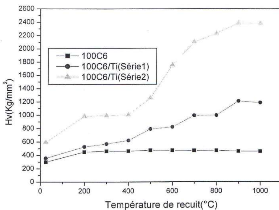
Figure 40: Variations de la microdureté avec la température de recuit des échantillons 100C6/Ti(série1, série2) et 100C6.
