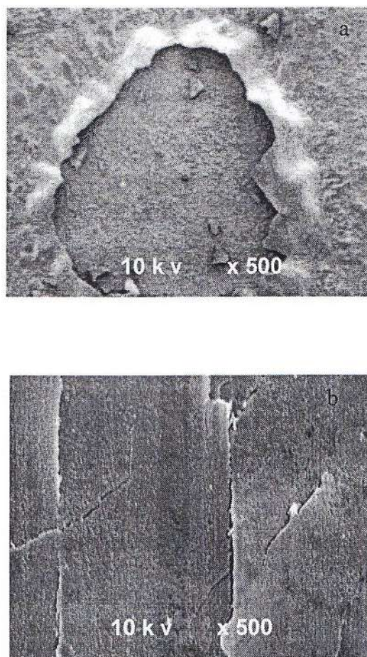
Figure 28: Etude morphologique avec MEB des échantillons 100C6/Ti, recuit à 1000°C x500 ; pendant 1h, série 1; (a) Gonflement puis détachement de la couche (b) fissuration puis détachement de la couche.
