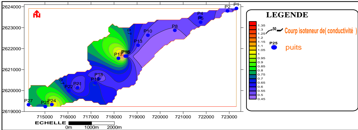
Fig.N°32 : Carte des teneurs en conductivité électrique ( \mu\text{S}/\text{Cm} ) de la nappe inféoflux.
