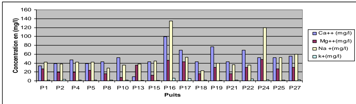
Fig N°.23: Histogrammes des cations de la nappe inféoflux.
