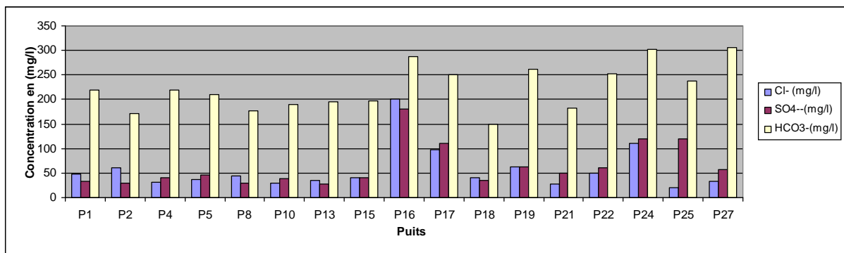
Fig. N°.24: Histogrammes des anions de la nappe inféoflux
