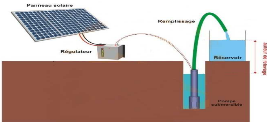
Pompe submersible - schéma de raccordement installation solaire
