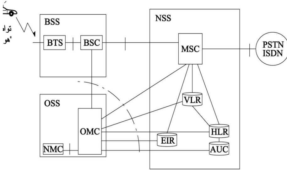
الشكل (1) بنية الشبكة الخلوية جي إس إم
