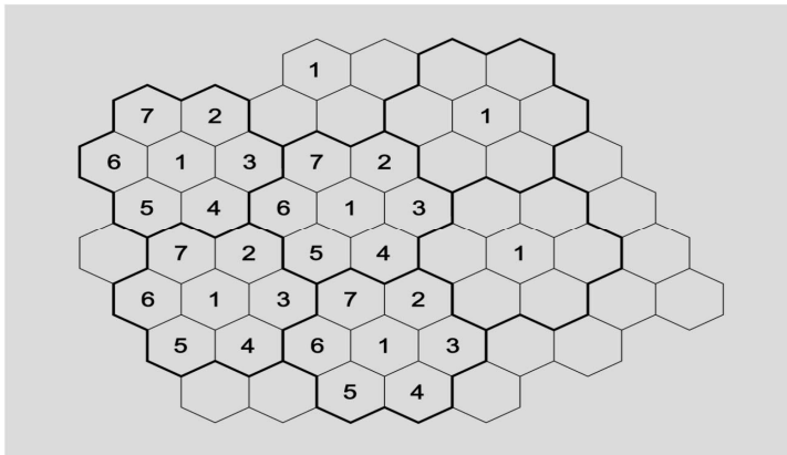
الشكل (3) مثال على بناء شبكة خلوية اعتماداً على سبع خلايا
