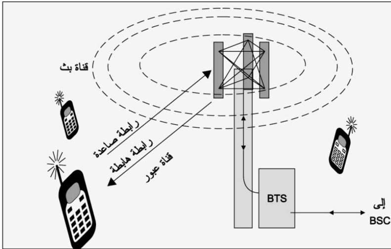
الشكل (2) خلية جي إس إم
